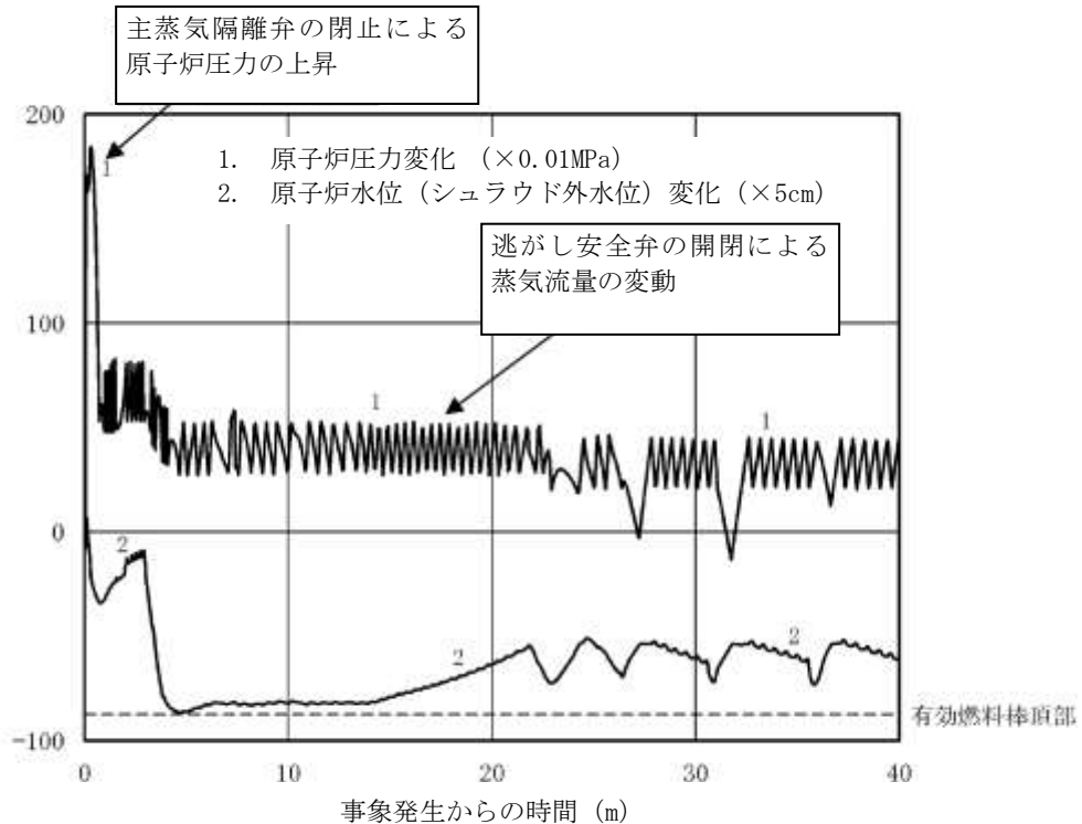
添付 8.2 図 原子炉停止機能喪失における原子炉圧力, 原子炉水位 (シュラウド外水位) の時間変化 (事象発生から 40 分後まで)
