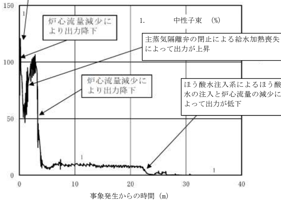
添付 8.1 図 原子炉停止機能喪失における中性子束の時間変化 (事象発生から 40 分後まで)
