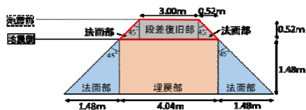
C-C' 断面
