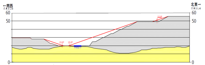
⑧断面
