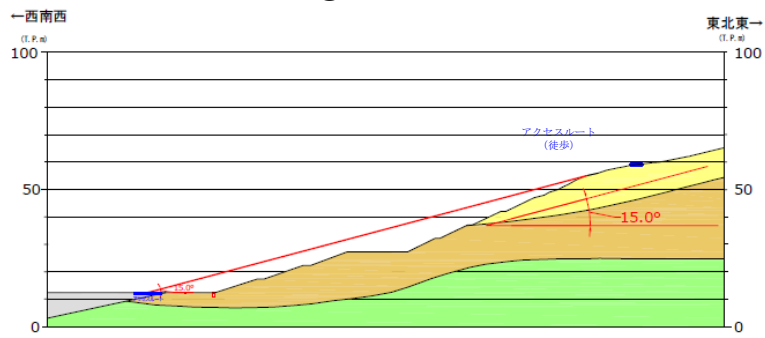
⑯断面
