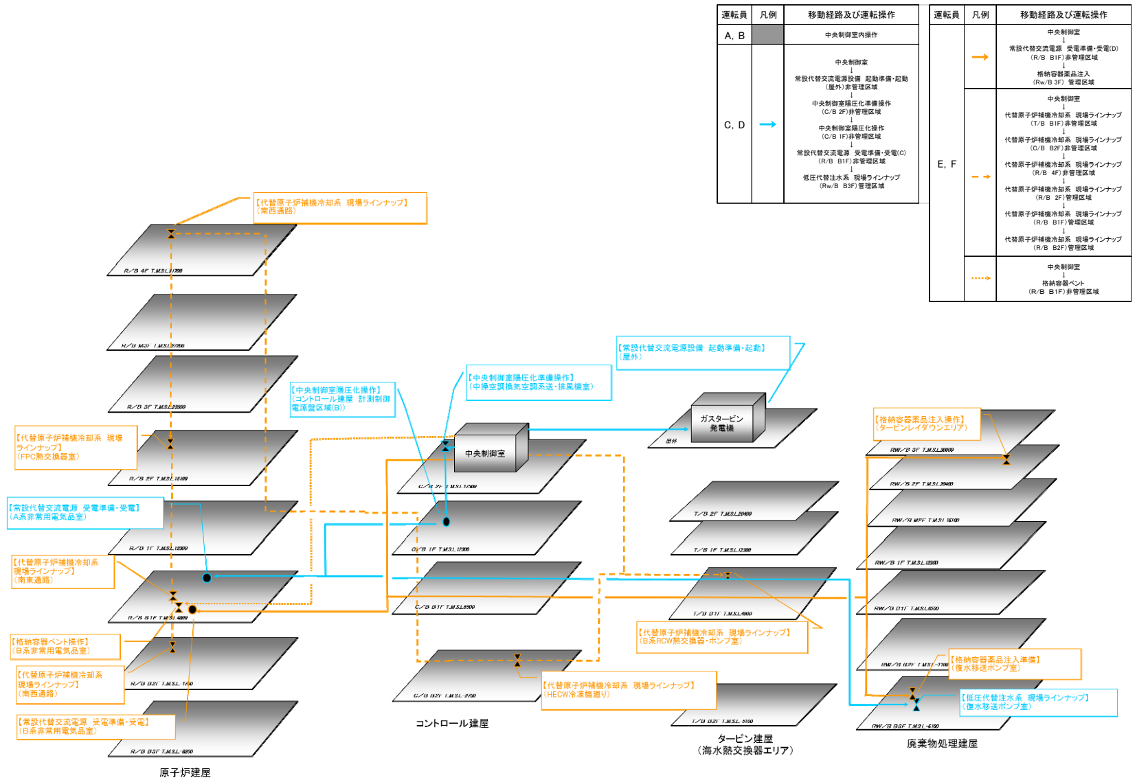
図 29-12 事故対象シーケンス：6号炉 格納容器過圧・加温破損（代替循環冷却なし）
