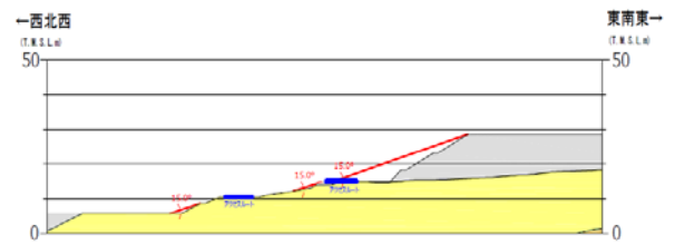
⑦断面
