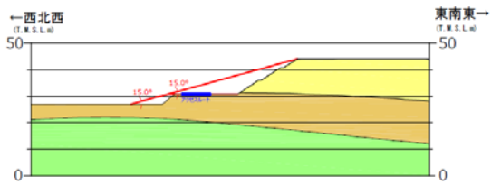
④断面
