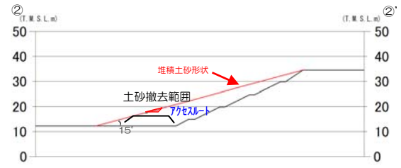
②-②' 断面図
