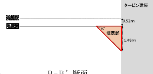
B-B' 断面
