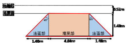
A-A' 断面
