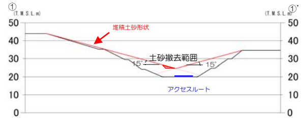
①-①' 断面図
