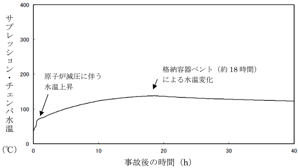
図 2.1.13 サプレッション・チェンバ水温の推移
