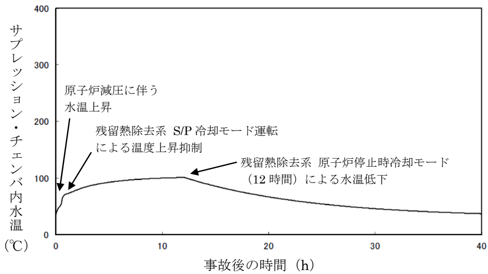
図 2.2.13 サプレッション・チェンバ水温の推移
