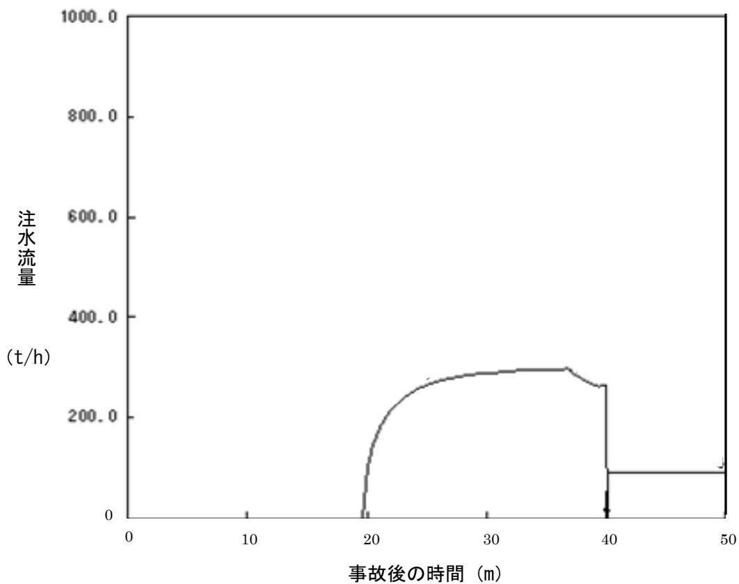
図 2.1.7 注水流量の推移
