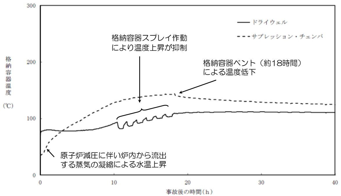
図 2.1.11 格納容器気相部の温度の推移
