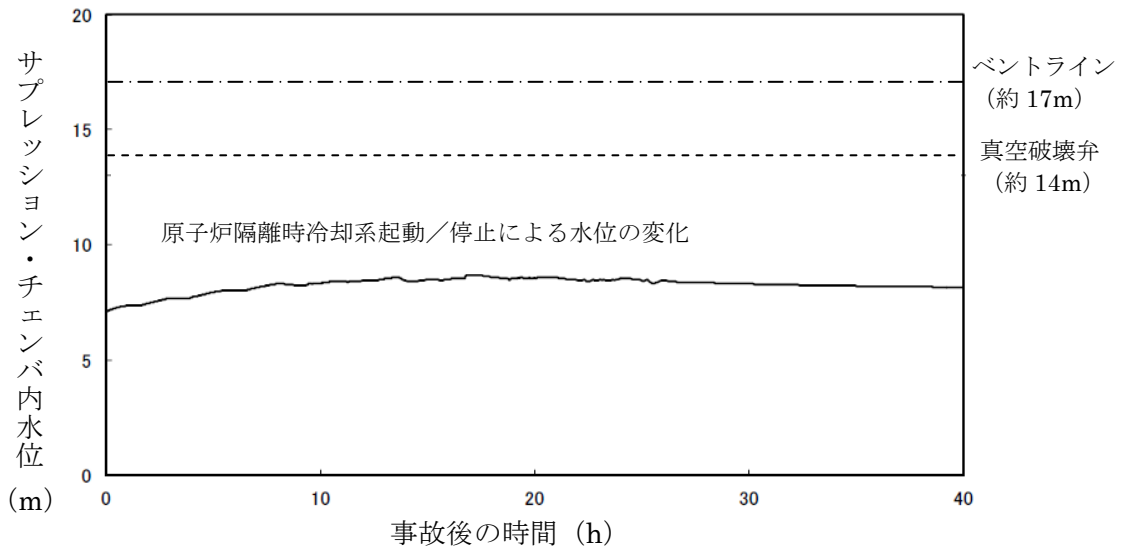
図 2.3.13 サプレッション・チェンバ水位の推移
