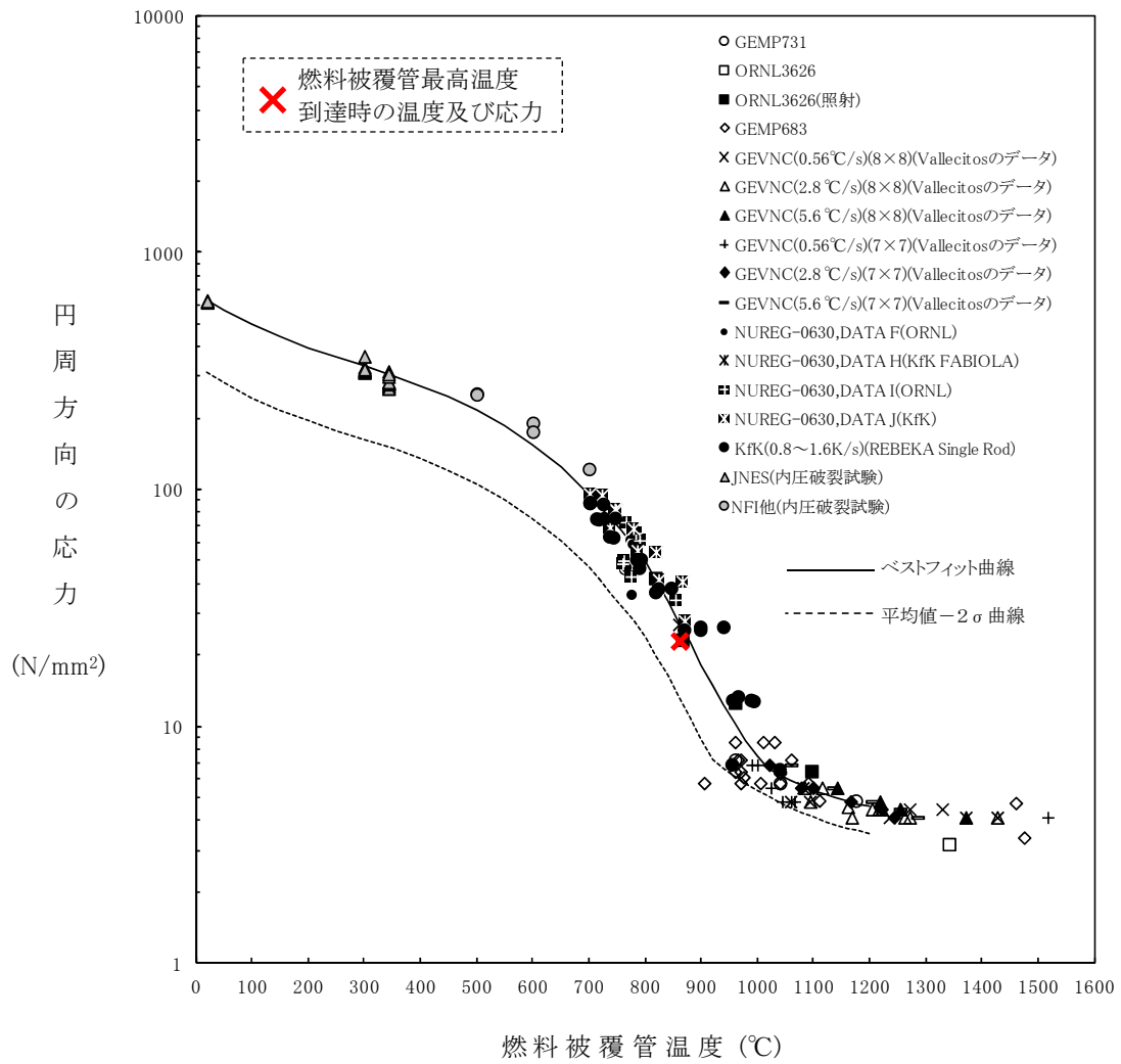
図 2.1.9 燃料棒に破裂が発生する時点の燃料被覆管温度と燃料被覆管の円周方向の応力の関係
