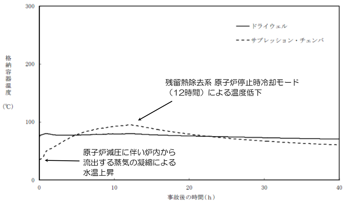
図 2.2.11 格納容器気相部の温度の推移
