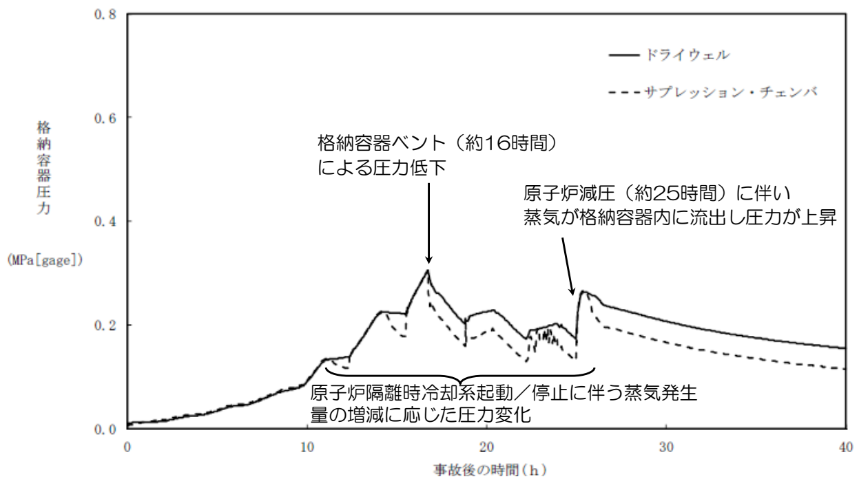
図 2.3.11 格納容器圧力の推移
