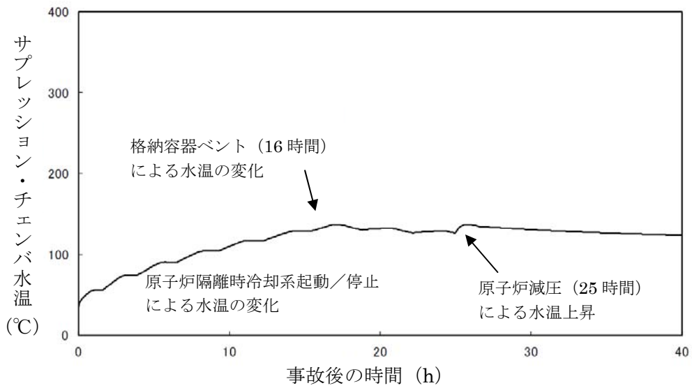
図 2.3.14 サプレッション・チェンバ水温の推移
