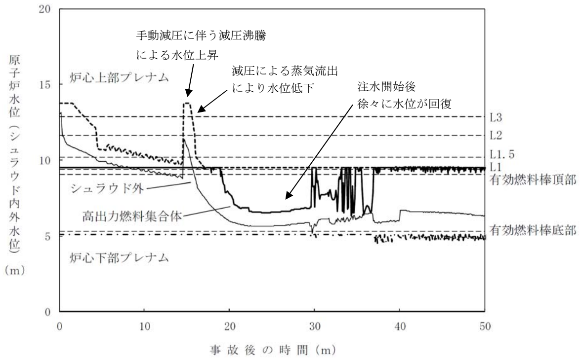
図 2.1.6 原子炉水位(シュラウド内外水位)の推移
