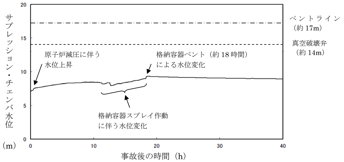
図 2.1.12 サプレッション・チェンバ水位の推移
