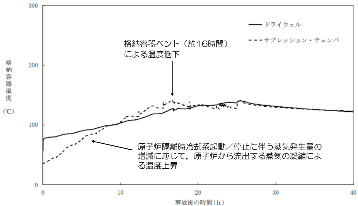
図 2.3.12 格納容器気相部の温度の推移
