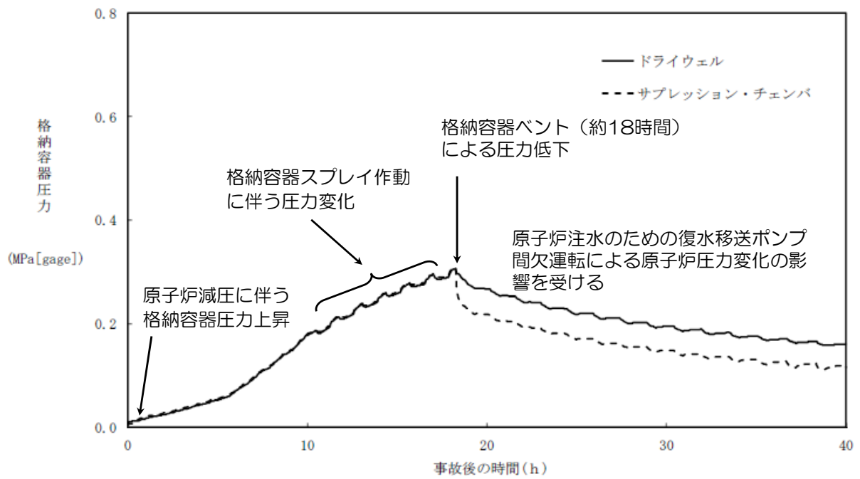
図 2.1.10 格納容器圧力の推移
