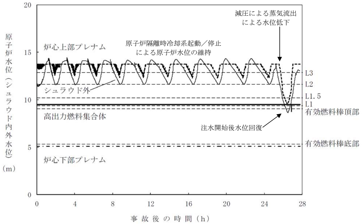
図 2.3.7 原子炉水位(シュラウド内外水位)の推移
