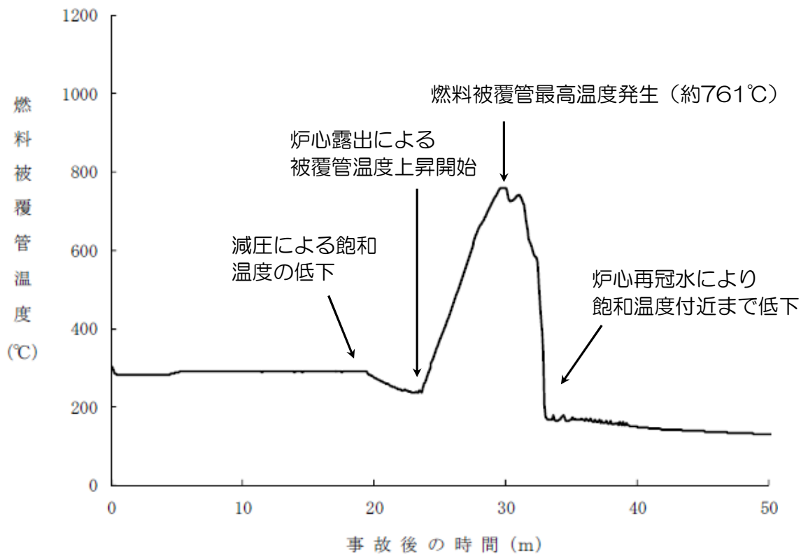
図 2.2.8 燃料被覆管温度の推移
