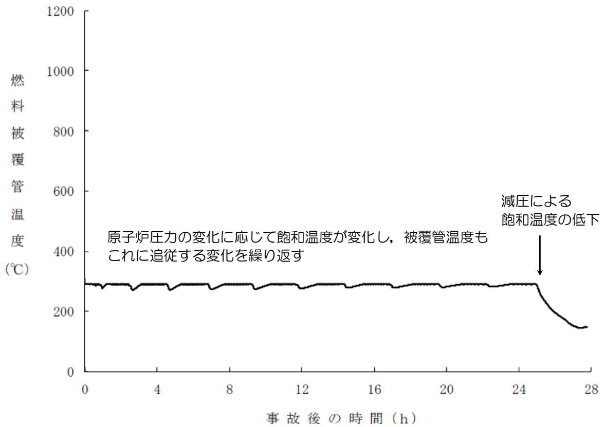
図 2.3.9 燃料被覆管温度の推移
