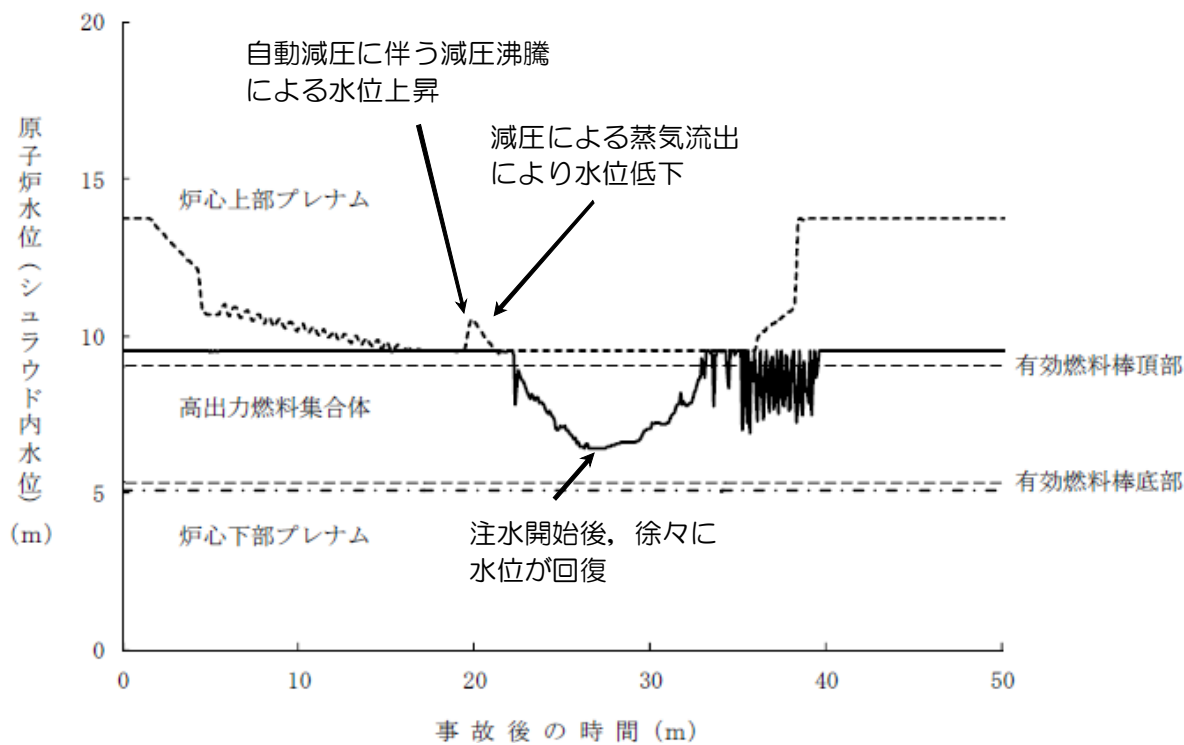
図 2.2.5 原子炉水位の推移
