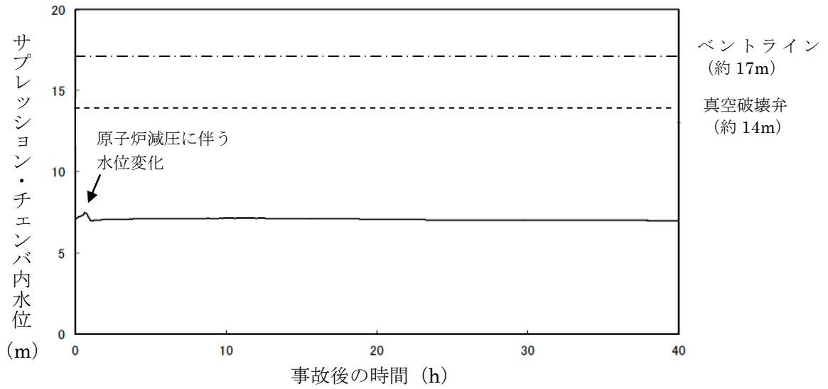
図 2.2.12 サプレッション・チェンバ水位の推移
