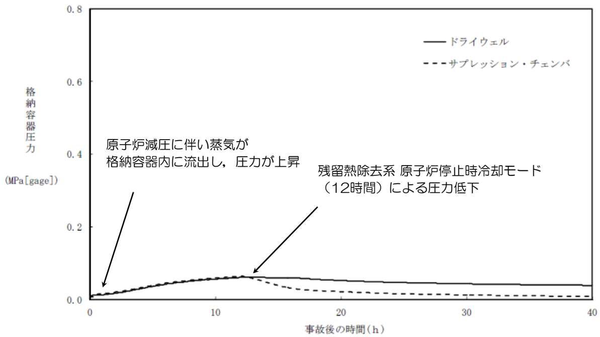
図 2.2.10 格納容器圧力の推移
