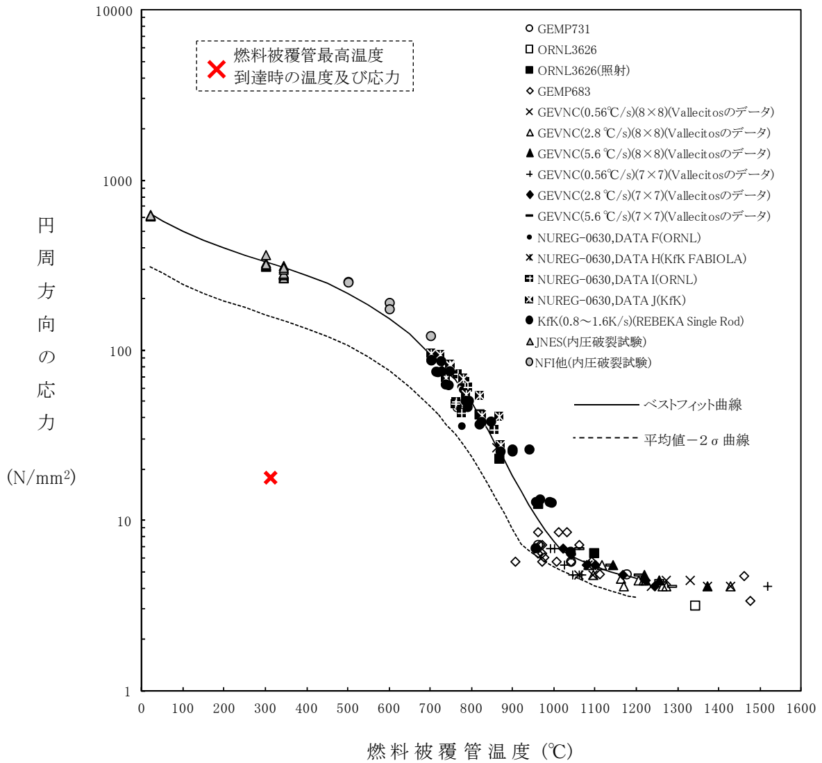
図 2.3.10 燃料棒に破裂が発生する時点の燃料被覆管温度と燃料被覆管の円周方向の応力の関係
