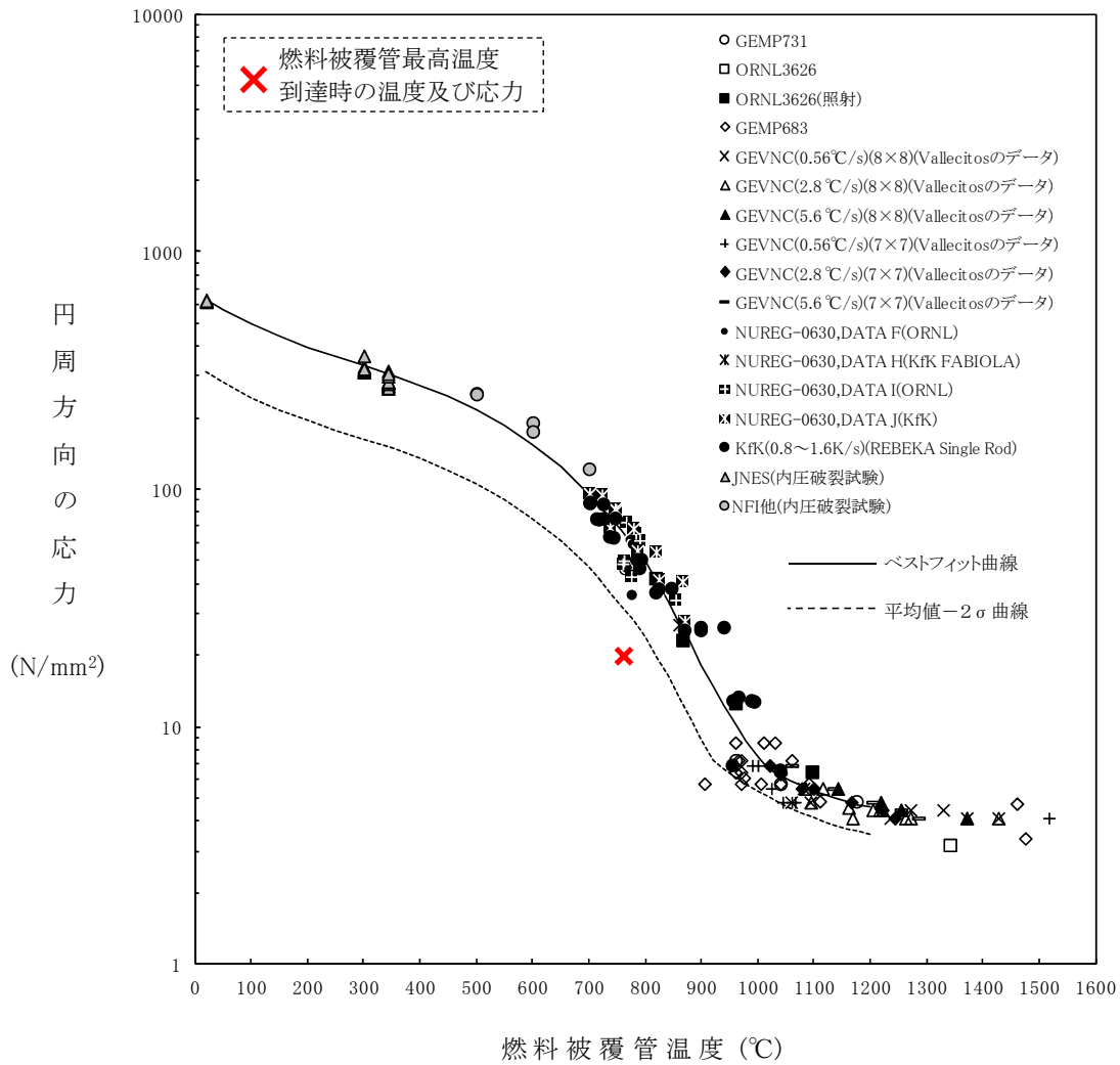
図 2.2.9 燃料棒に破裂が発生する時点の燃料被覆管温度と燃料被覆管の円周方向の応力の関係
