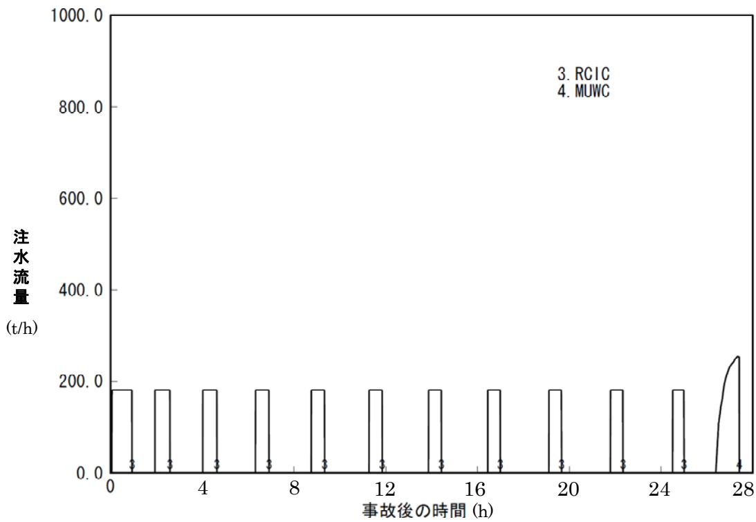
図 2.3.8 注水流量の推移
