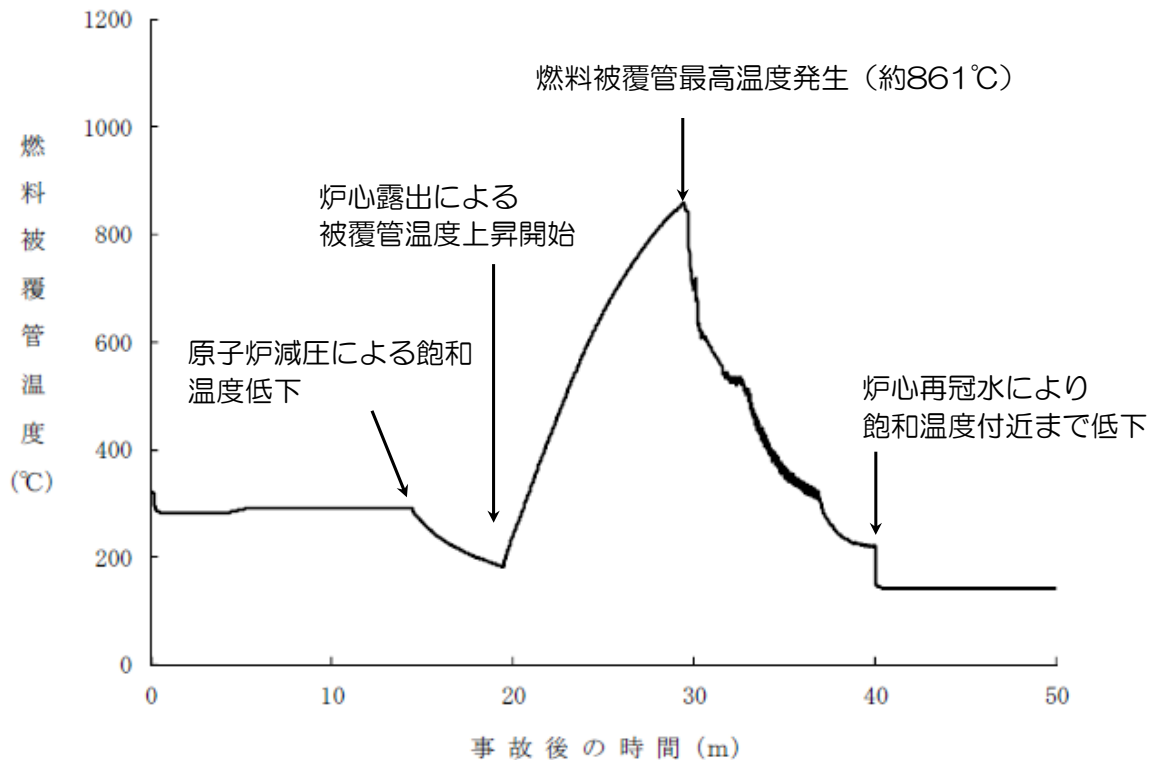
図 2.1.8 燃料被覆管温度の推移
