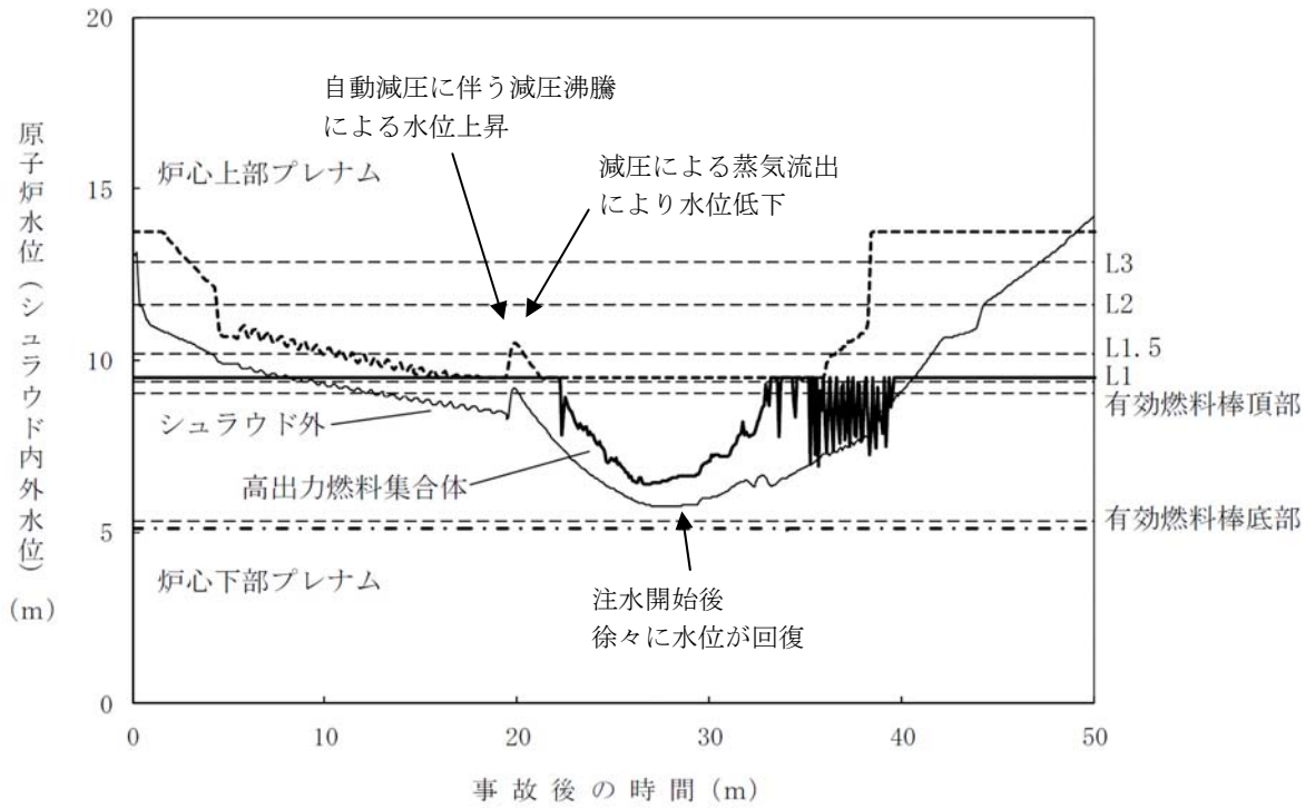
図 2.2.6 原子炉水位(シュラウド内外水位)の推移
