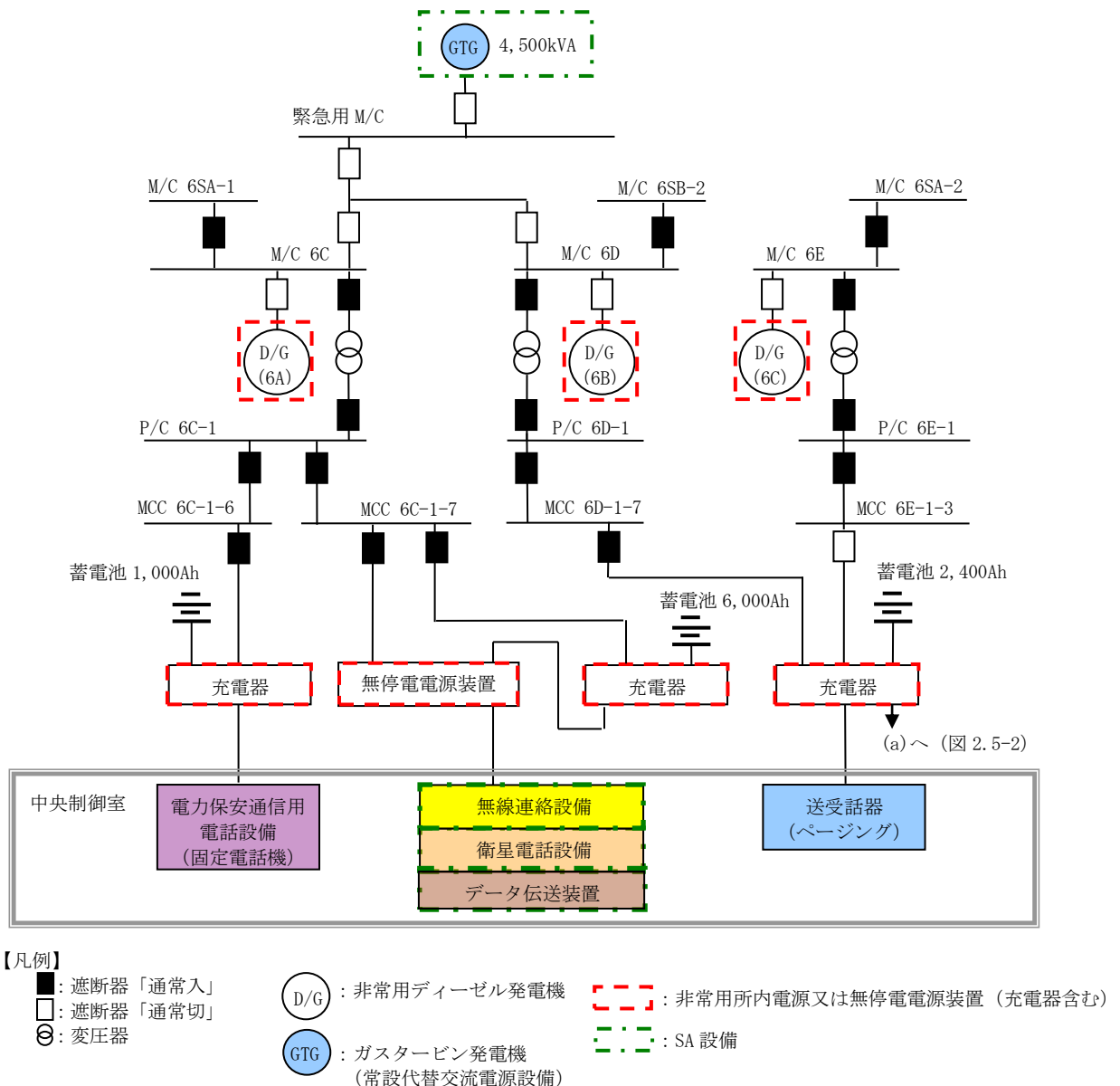
図2.5-1 中央制御室における通信連絡設備の電源構成（6号炉）
