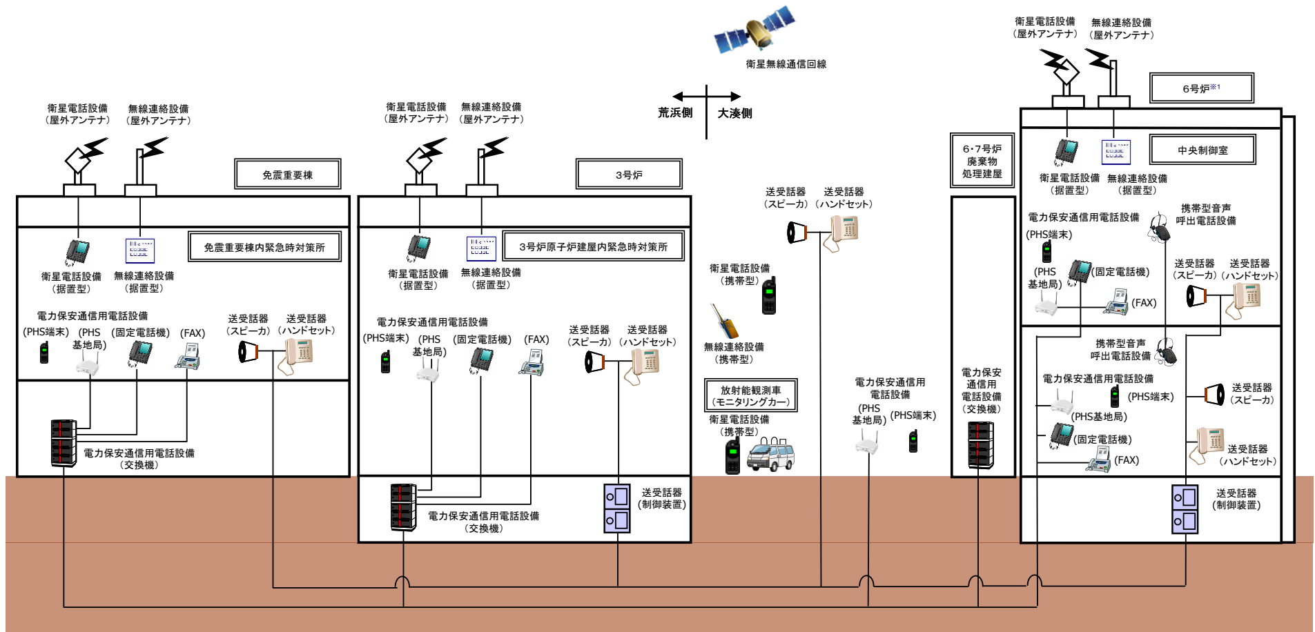
図2.1-1 通信連絡設備（発電所内）の概要 [通信連絡設備（発電所外）と共用を含む]
