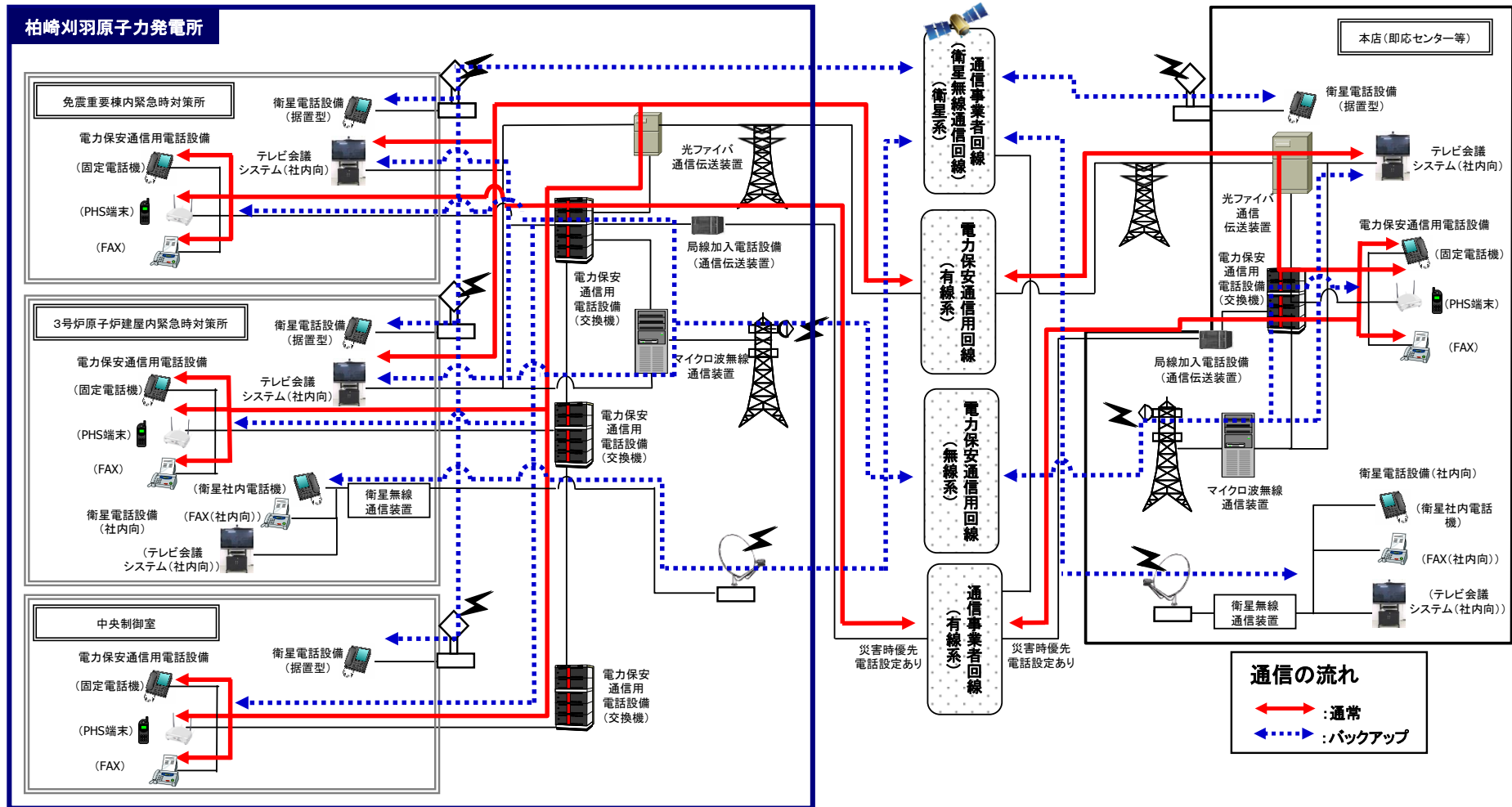
図2.2-1 通信連絡設備（発電所外〔社内関係箇所〕）の概要 （電力保安通信用電話設備，局線加入電話設備，衛星電話設備，テレビ会議システム（社内））
