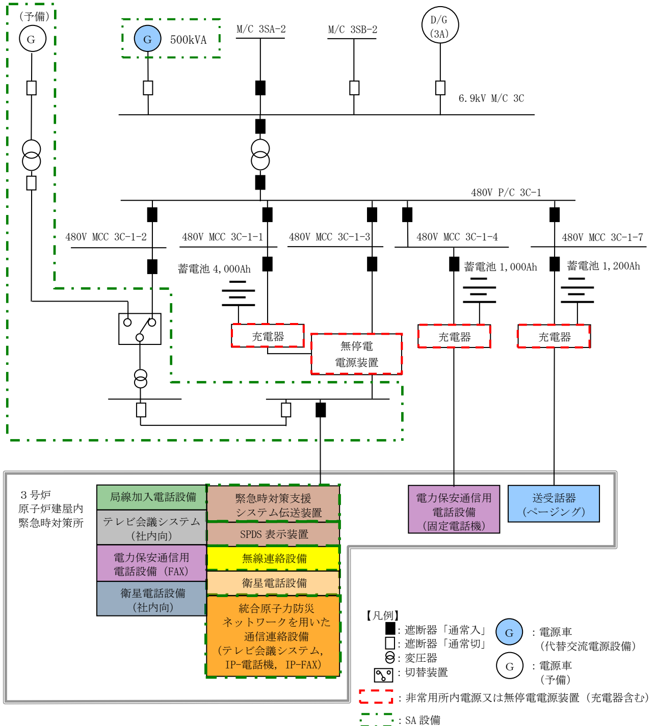
図2.5-4 3号炉原子炉建屋内緊急時対策所における通信連絡設備の電源構成
