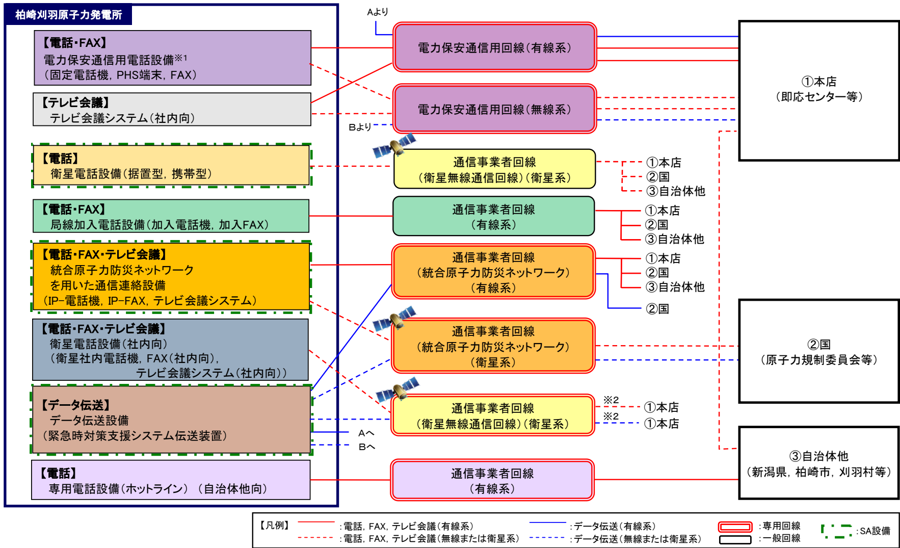
図2. 4-1 多様性を確保した通信回線の概要
