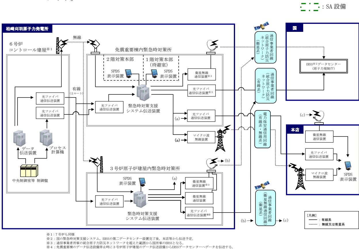
図2.3-1 データ伝送設備の概要
