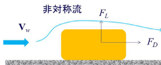
図 9(b) 地面付近で飛来物へ作用する力
