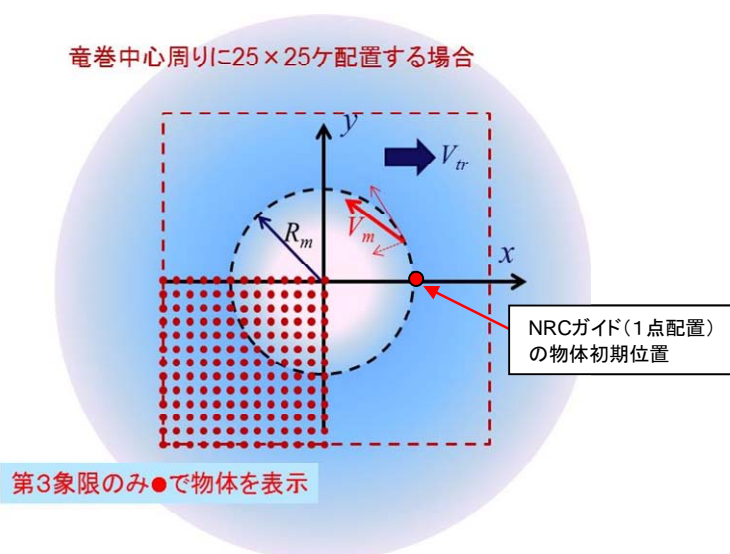
図 10 飛来物評価における竜巻と物体の位置関係
