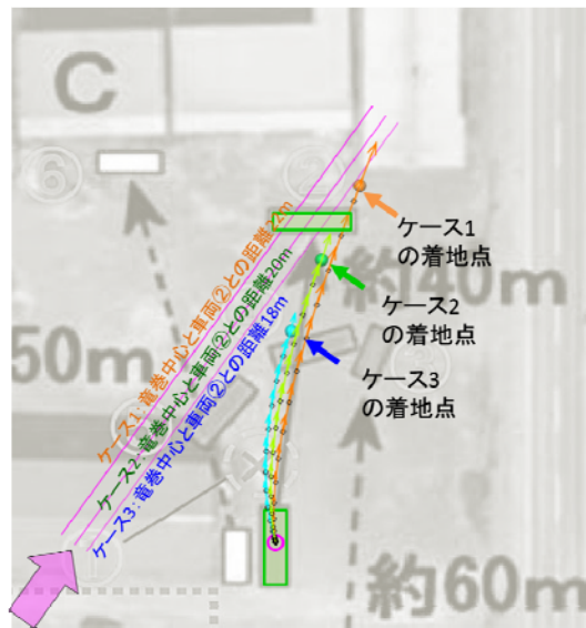
図 16 フジタモデルによるトラック飛散の再現解析結果
