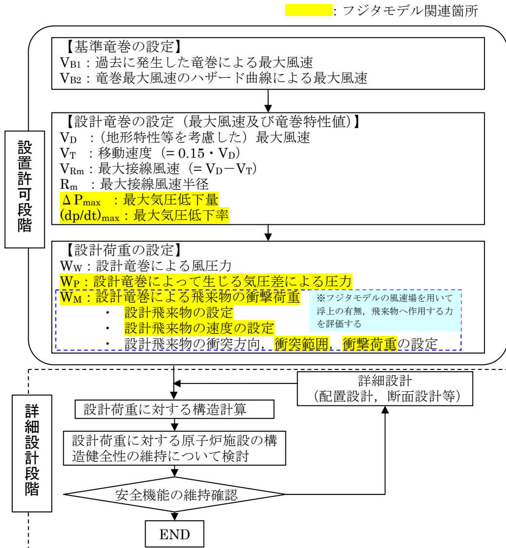
図1 竜巻影響評価フローとフジタモデルの関連箇所
