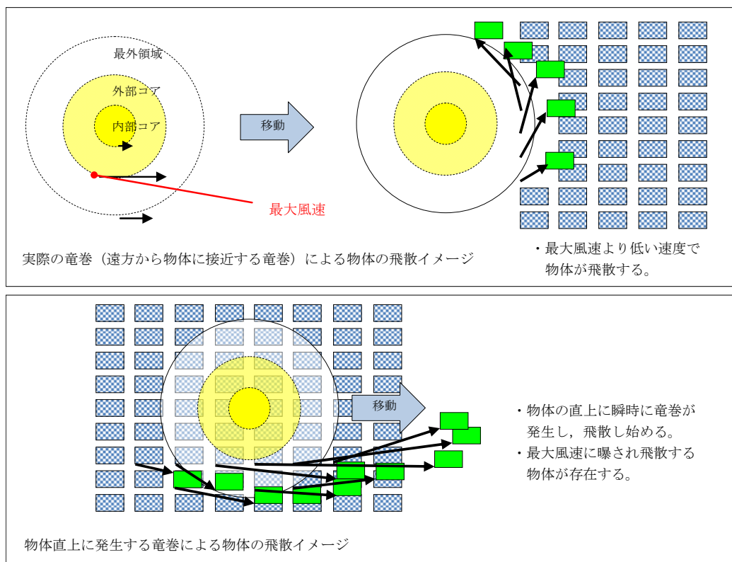
図 12 物体に接近する竜巻と物体直上に発生する竜巻の比較イメージ図
