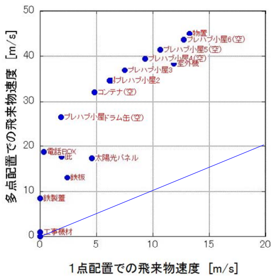
図 11 1点配置時と多点配置時の最大飛来物速度の比較 (左) と物体のパラメータ (右)
