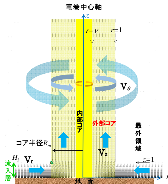
図4 フジタモデルの概要
