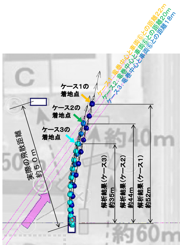
図17 フジタモデルによる乗用車飛散の再現解析結果
