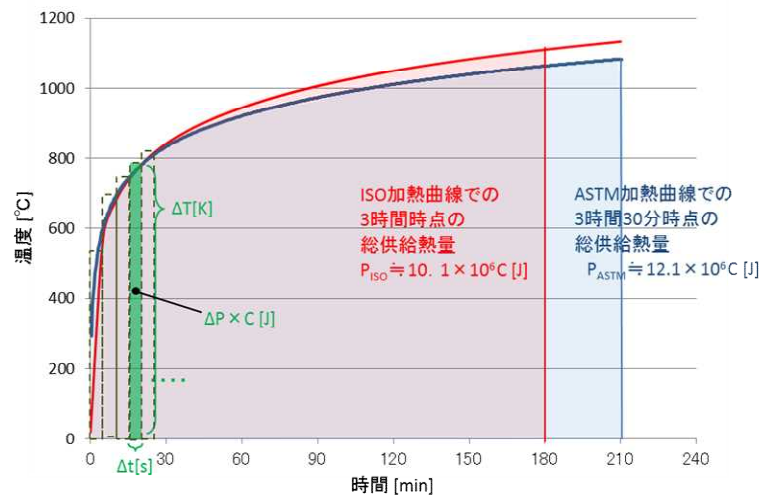
図1 ASTM加熱曲線とISO加熱曲線の総供給熱量の比較
