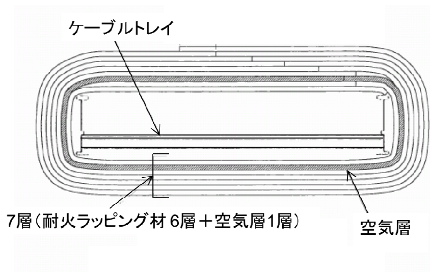
図 14 耐火ラッピング施工時のケーブルトレイ断面図
