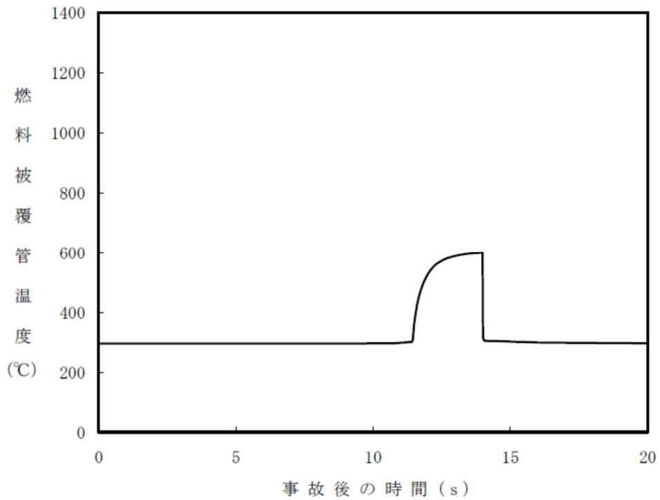
図 6-5 給水制御系故障解析結果 (T/B 建屋起因) (2/2)
