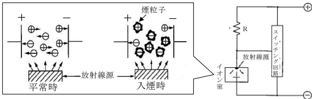
図 2 : イオン化式煙感知器概要
