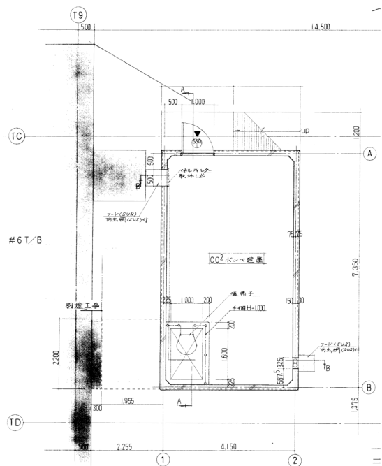
(a) 平面図
