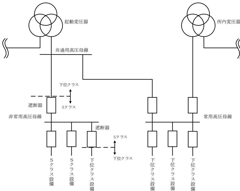
受電系統概念図
