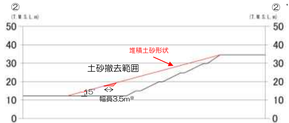
②—② ‘断面図
