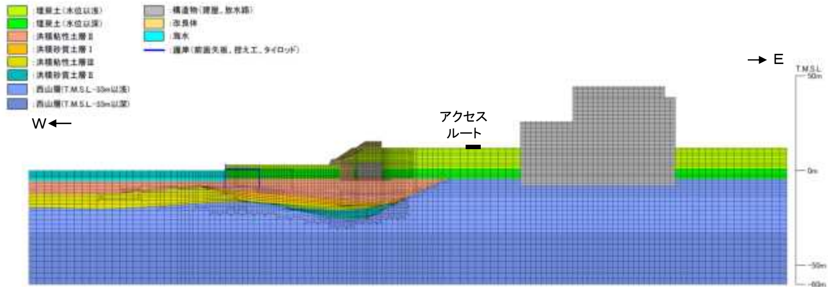
解析モデル図
