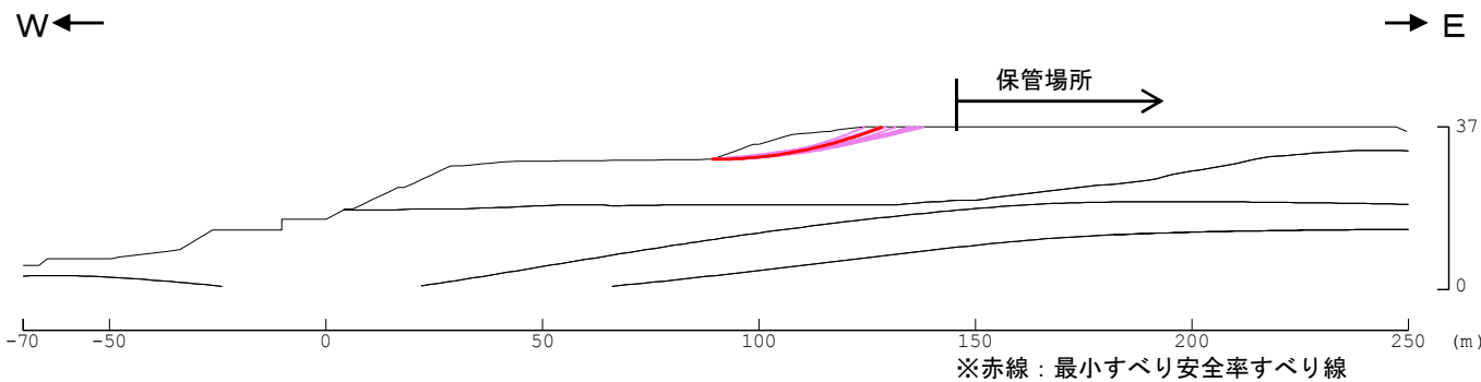
すべり安全率が1を下回るすべり線
