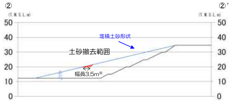
②-②'断面図
