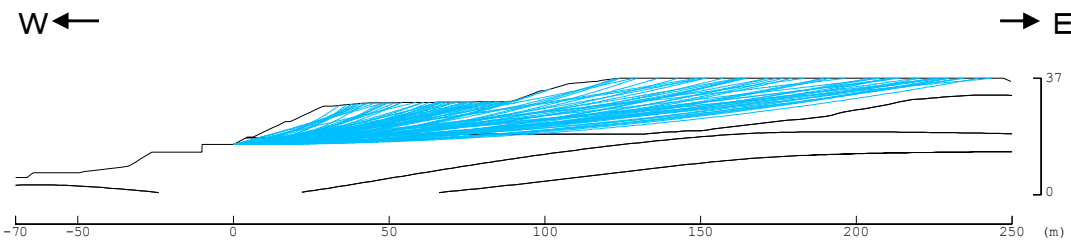
すべり安全率を算出したすべり線①
