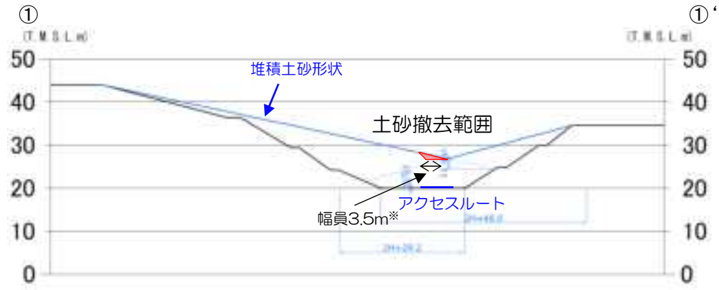
①-①'断面図
