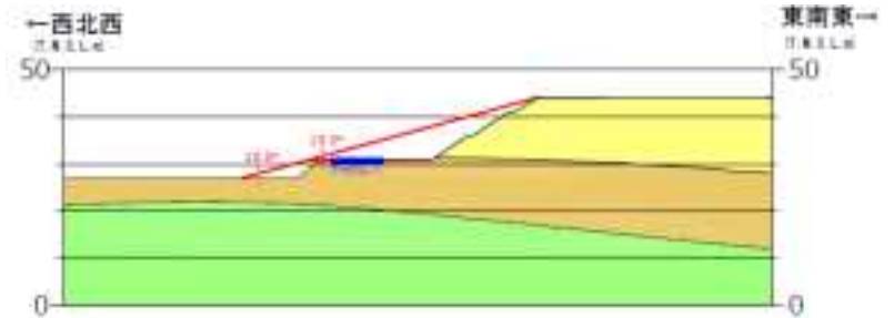
⑤断面
