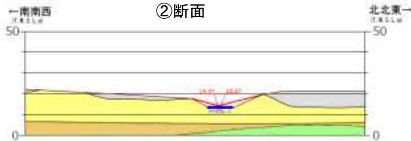
③断面
