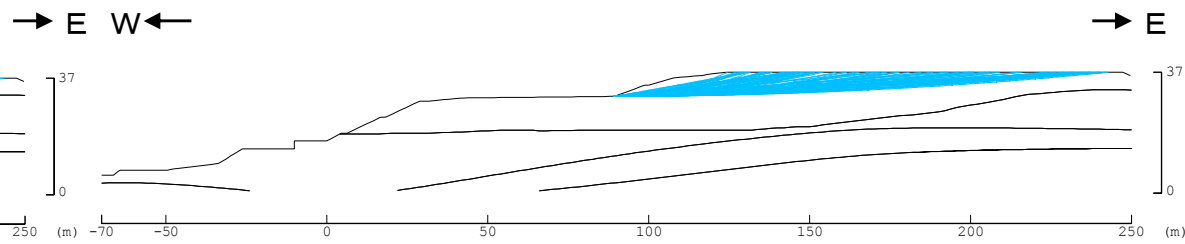
すべり安全率を算出したすべり線②
