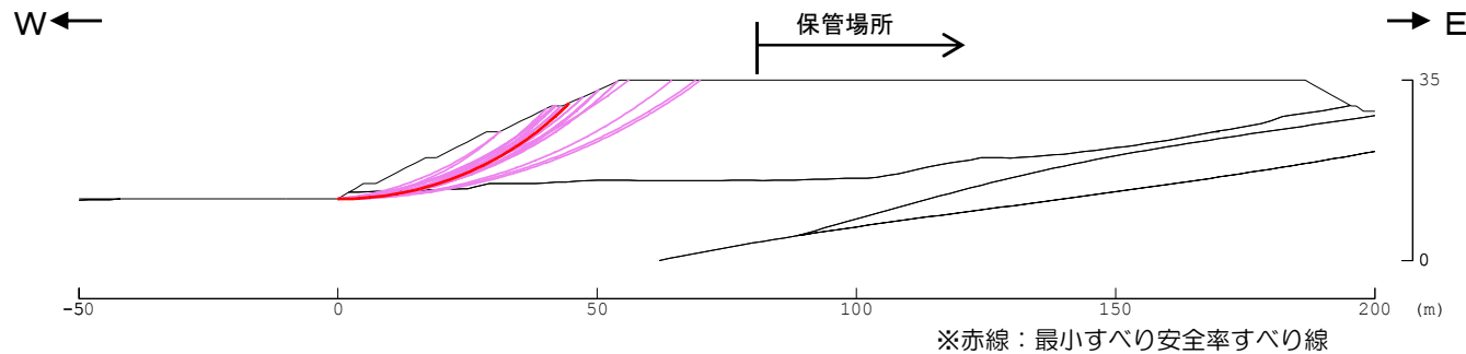
すべり安全率が1を下回るすべり線
