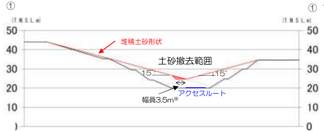
①—① ‘断面図
