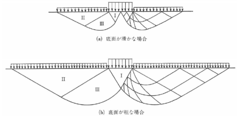
図 10.10 一般的なすべり面の形状
