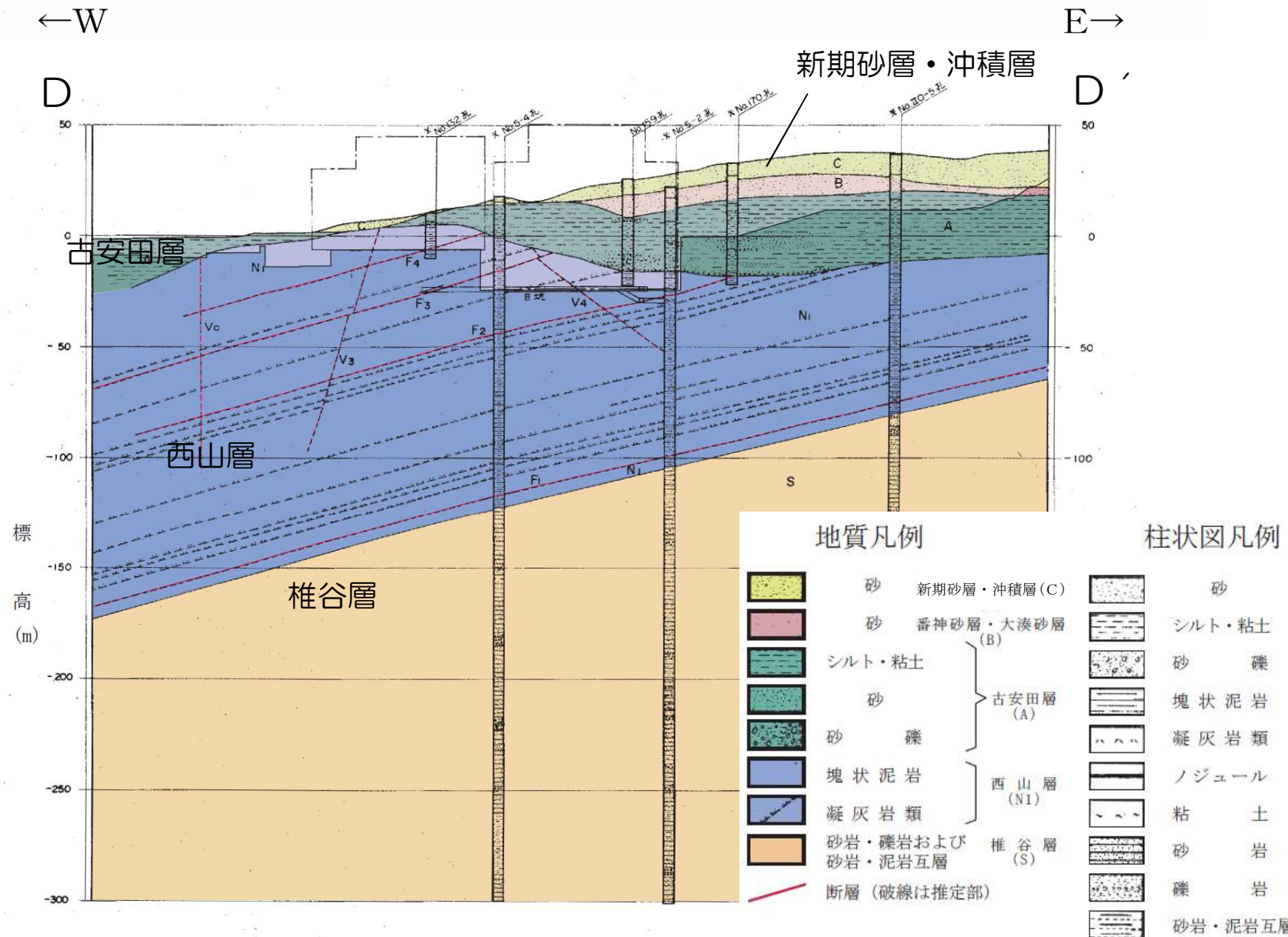
地質断面図 (D—D')
