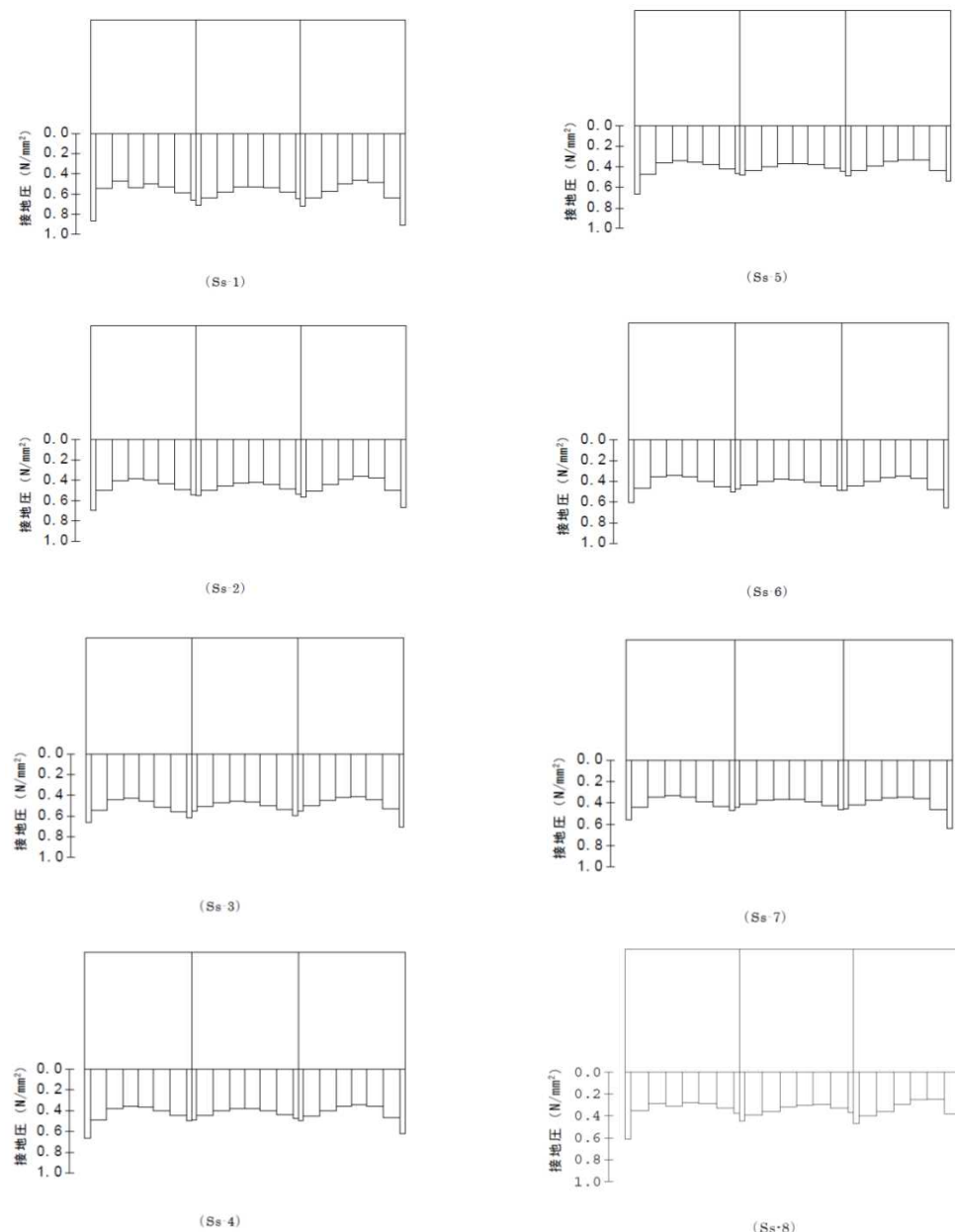
接地圧分布図（鉛直力最大時）
