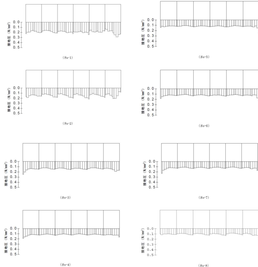
接地圧分布図（鉛直力最大時）
