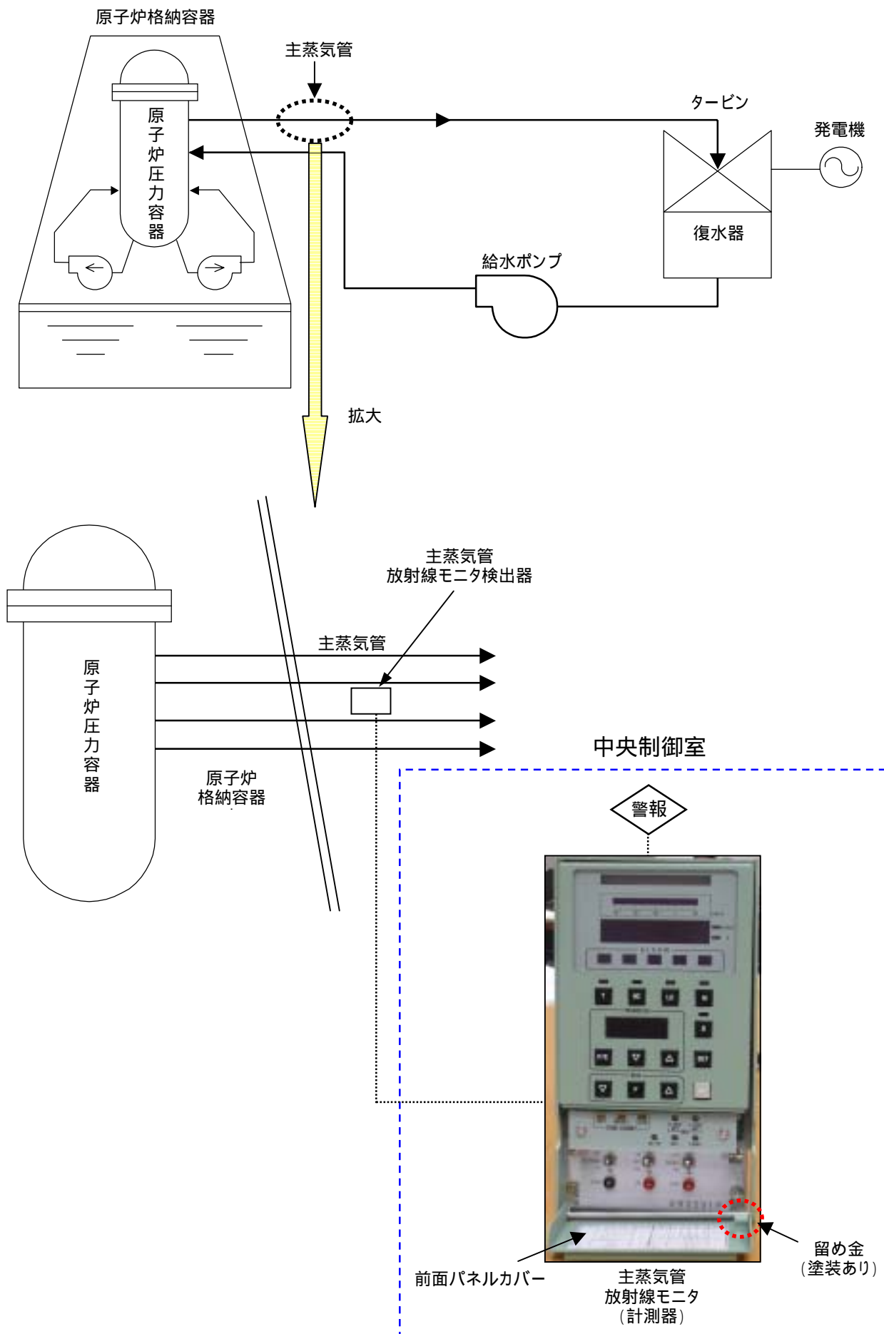
主蒸気管放射線モニタ 概略系統図
