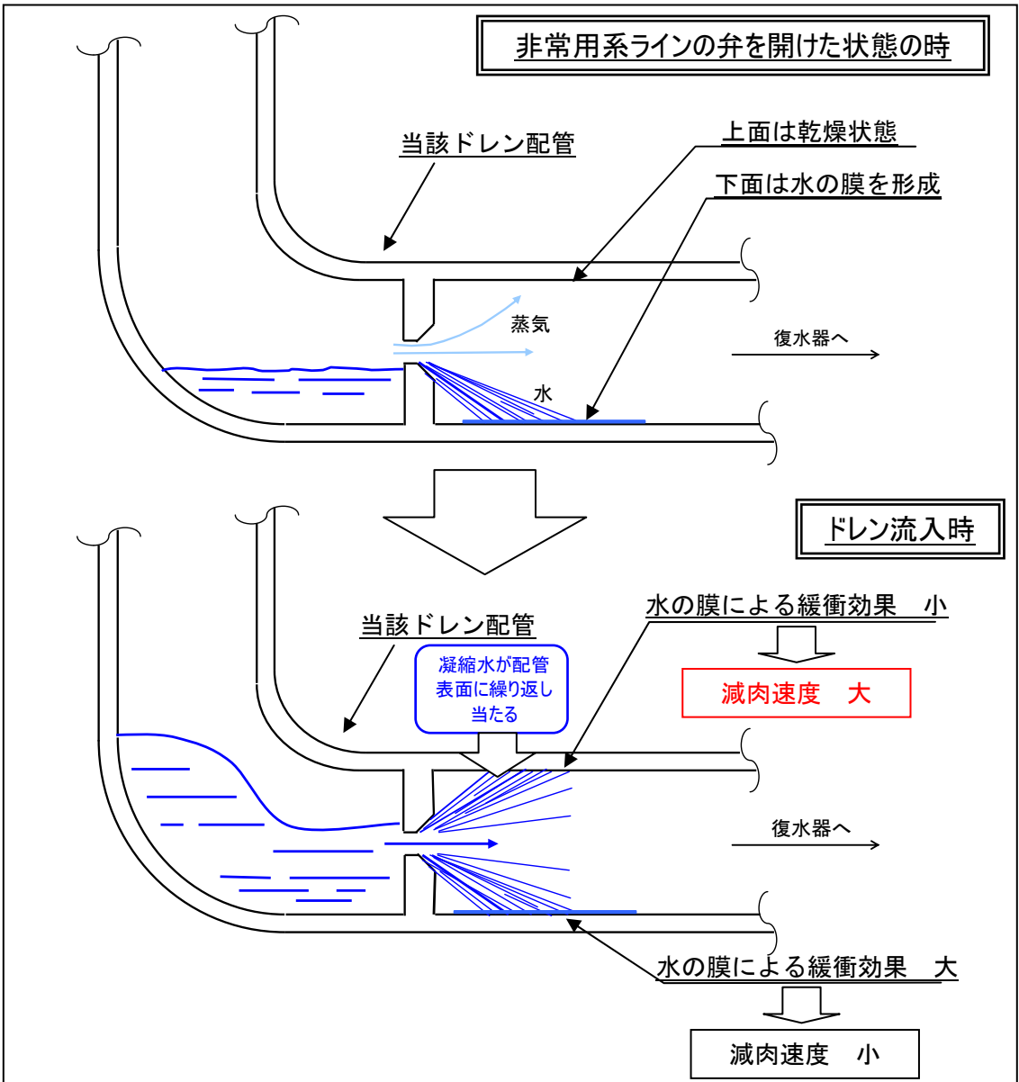
常用系ライン オリフィス近傍の侵食進捗 イメージ図
