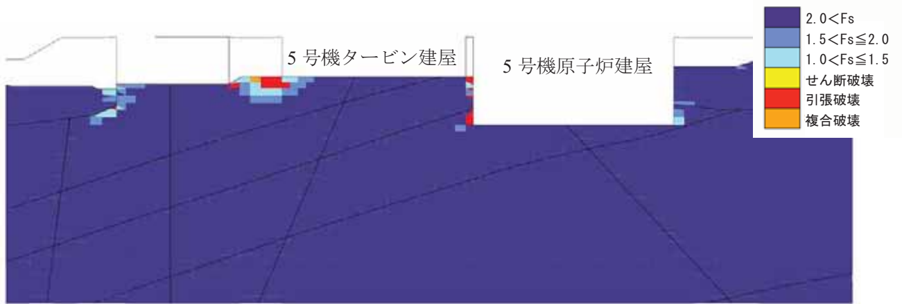
要素ごとの安全係数
