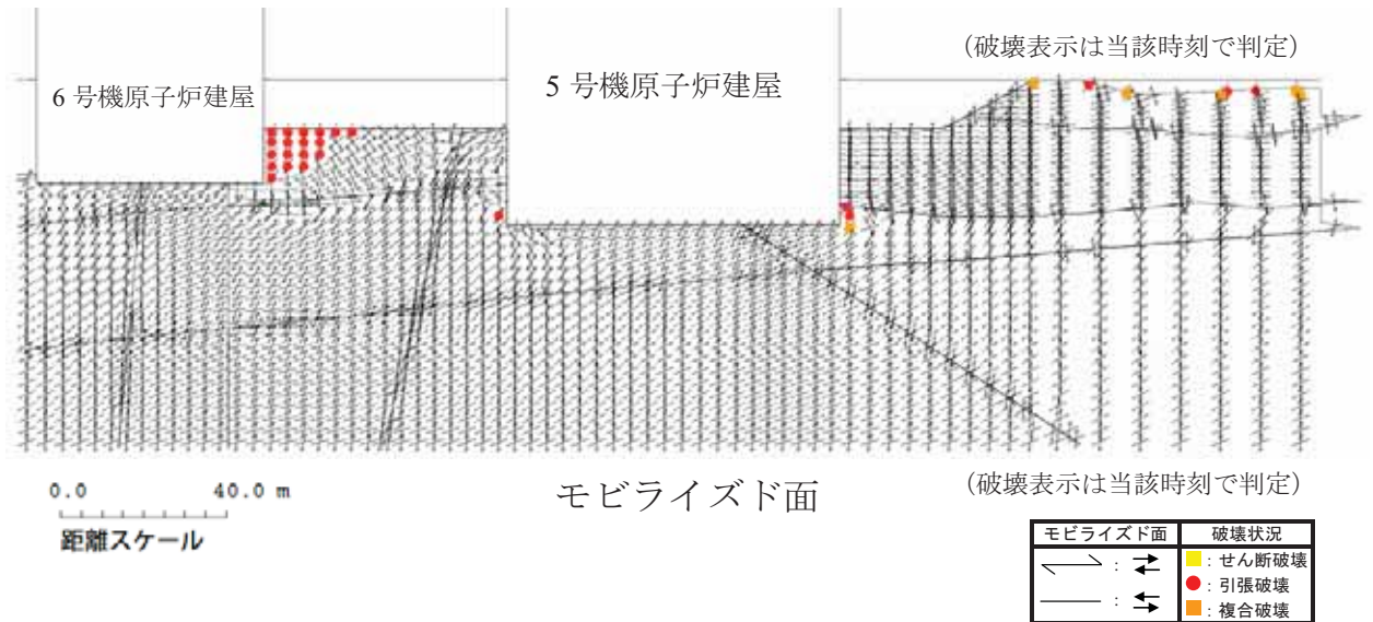
第 5.3.3-1 図(1) 要素ごとの安全係数およびモビライズド面 (原子炉建屋基礎地盤，汀線平行断面，Ss-1，要素鉛直応力最大時，T=6.77 秒)
