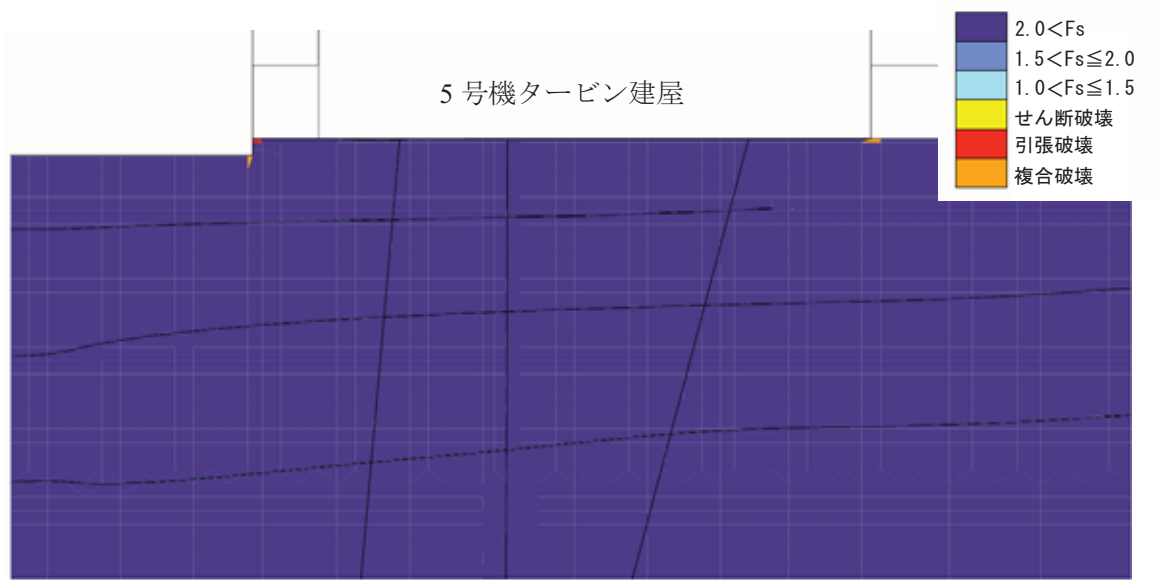
要素ごとの安全係数
