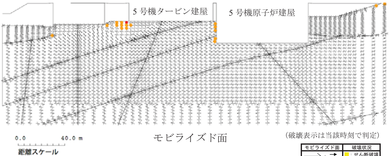
第 5.3.3-2 図(3) 要素ごとの安全係数およびモビライズド面
