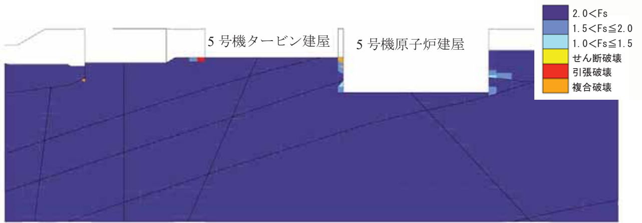
要素ごとの安全係数
