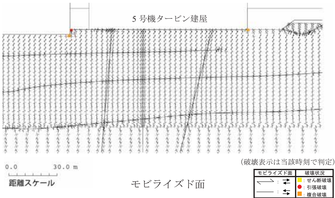
第 5.3.3-2 図(2) 要素ごとの安全係数およびモビライズド面
