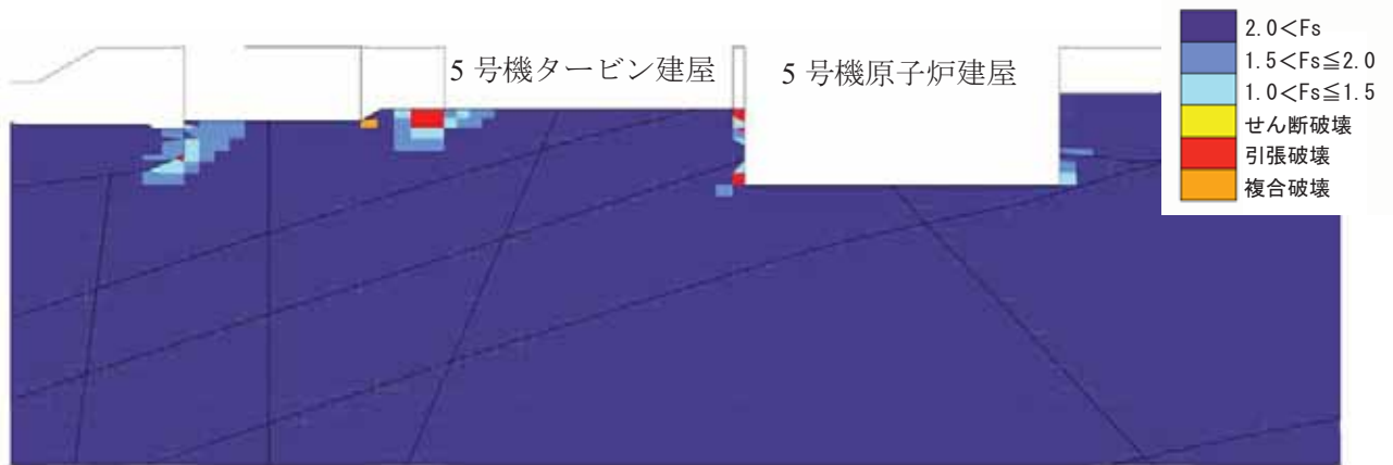
要素ごとの安全係数
