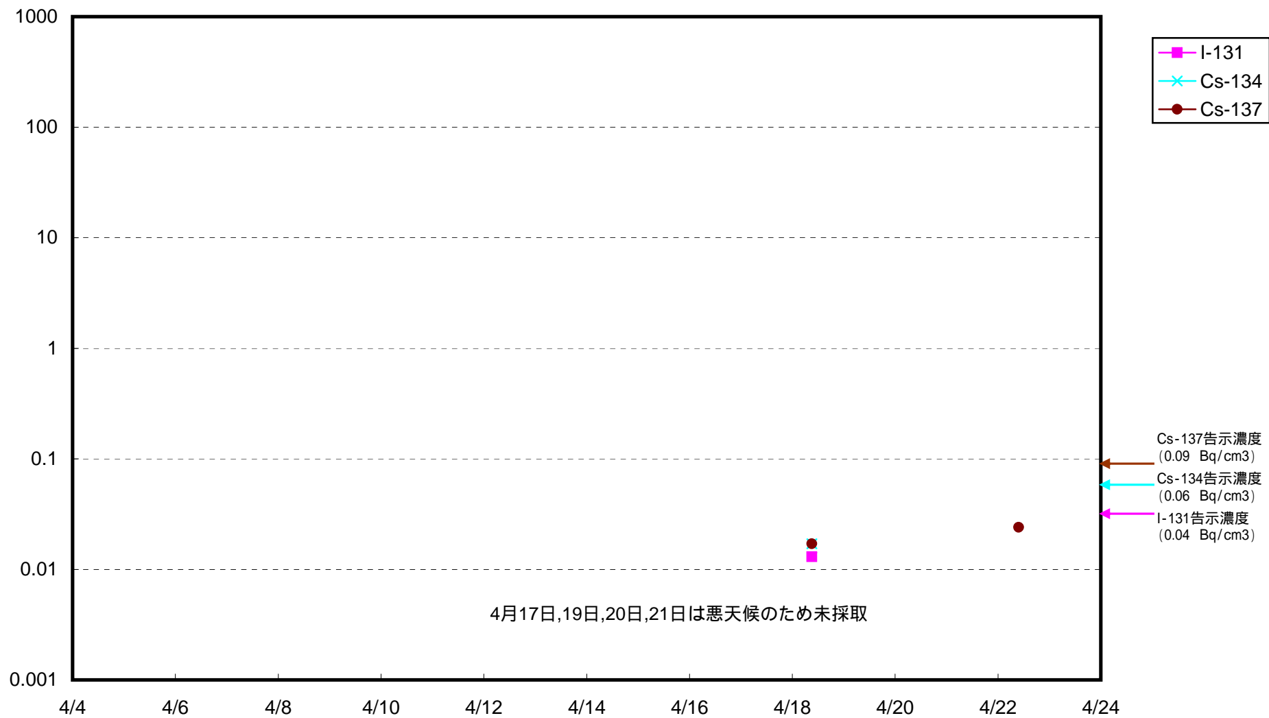
小高区沖合8km付近 海水放射能濃度 (Bq / cm 3 )
