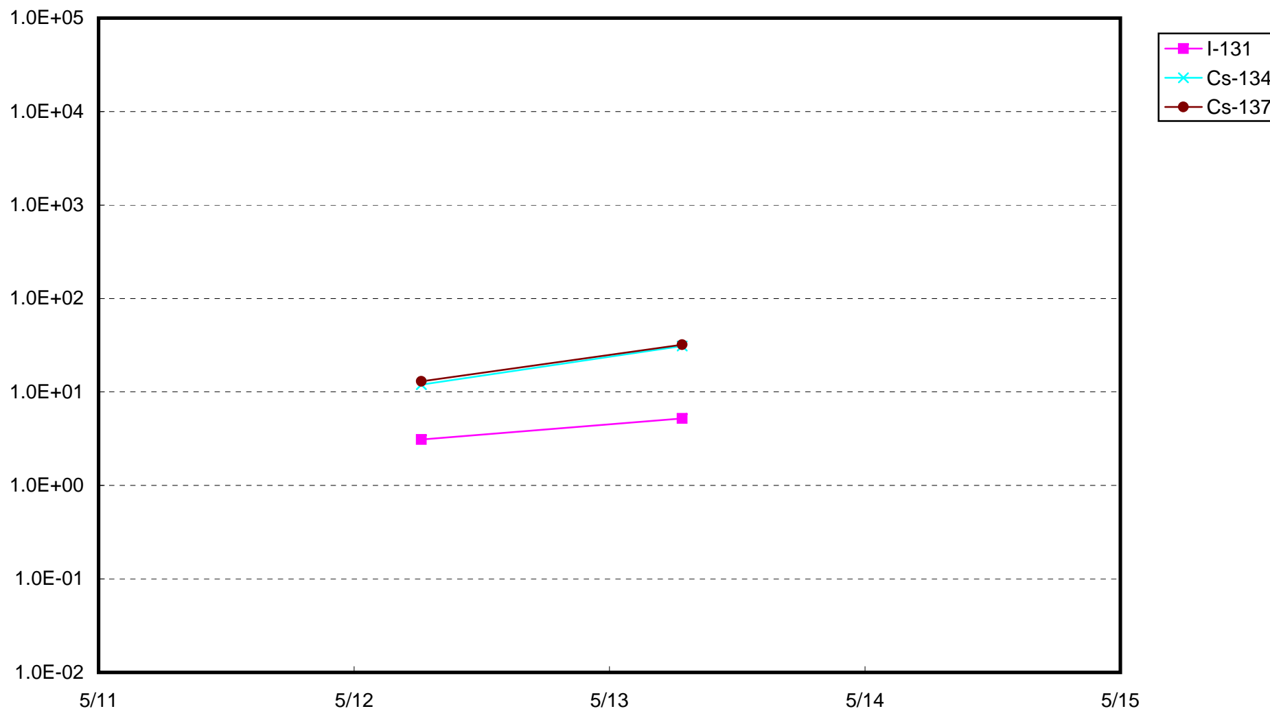
福島第一 1号機バースクリーン付近海水放射能濃度(シルトフェンス外側) (Bq / cm 3 )
