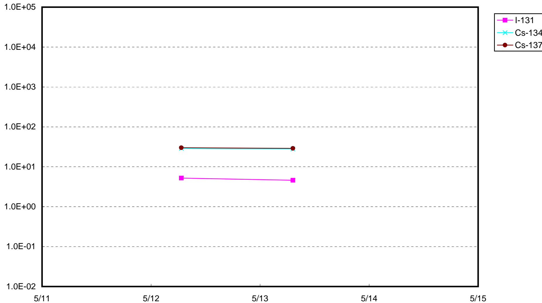
福島第一 4号機バースクリーン付近海水放射能濃度(シルトフェンス外側) (Bq / cm 3 )
