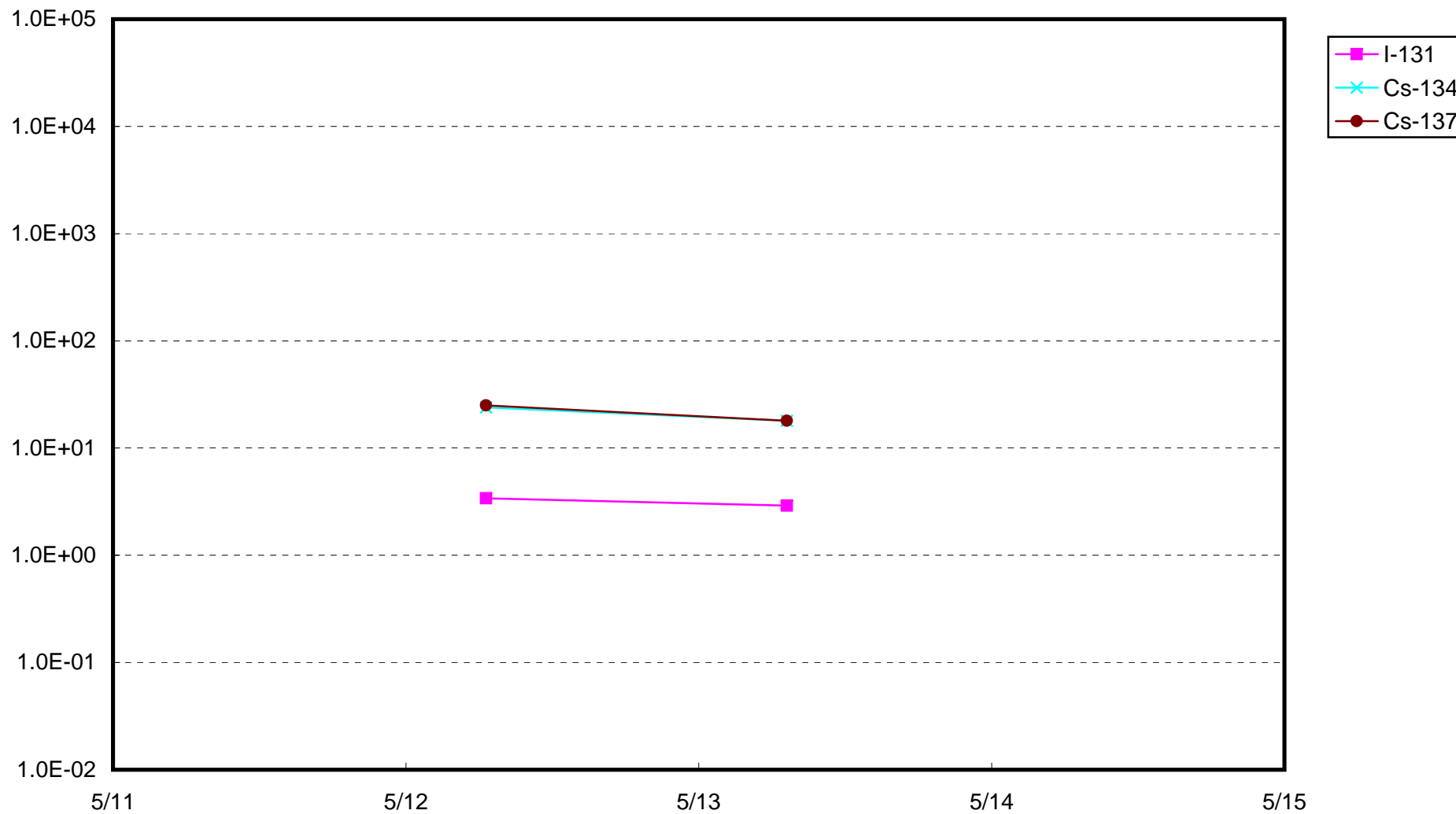
福島第一 4号機バースクリーン付近海水放射能濃度(シルトフェンス内側) (Bq / cm 3 )
