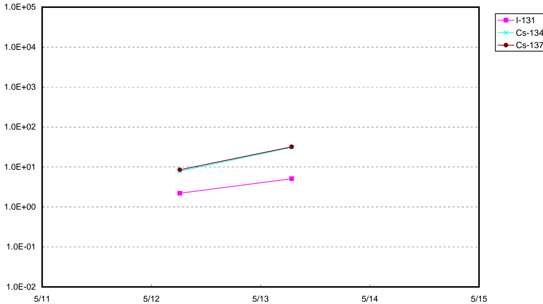
福島第一 1号機バースクリーン付近海水放射能濃度(シルトフェンス内側) (Bq / cm 3 )
