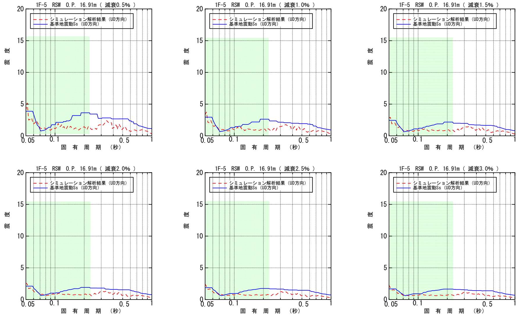
図-4.4.3.12 原子炉遮へい壁 O.P. 16.91m 床応答スペクトル (鉛直方向)
