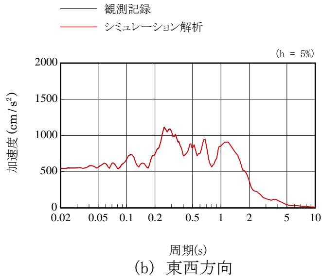
参図-3.2 5号機原子炉建屋基礎版上の加速度応答スペクトルの比較 観測記録 (5-R2) とシミュレーション解析結果に基づく応答波
