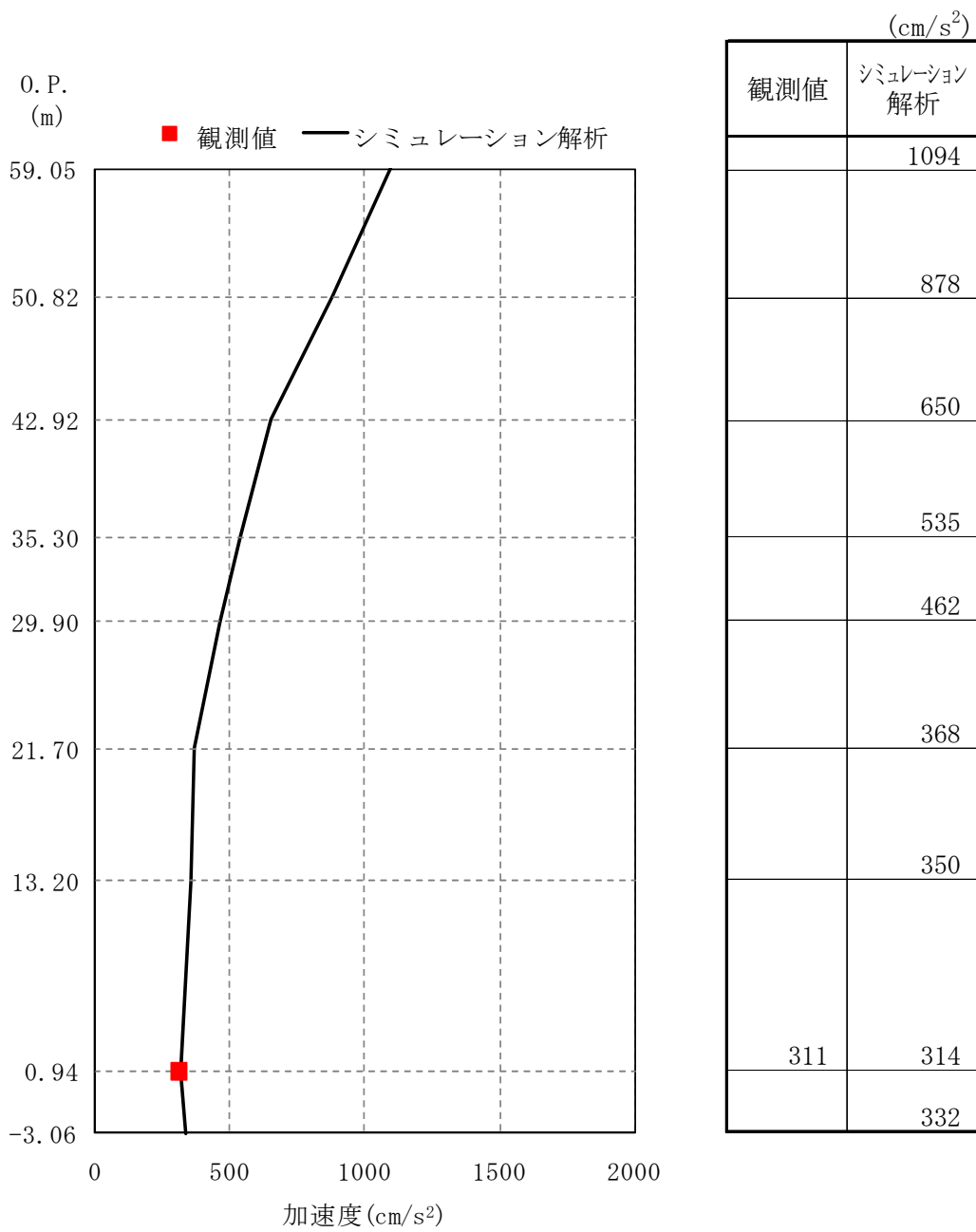
図-3.5.1(1) 最大応答加速度 (南北方向)
