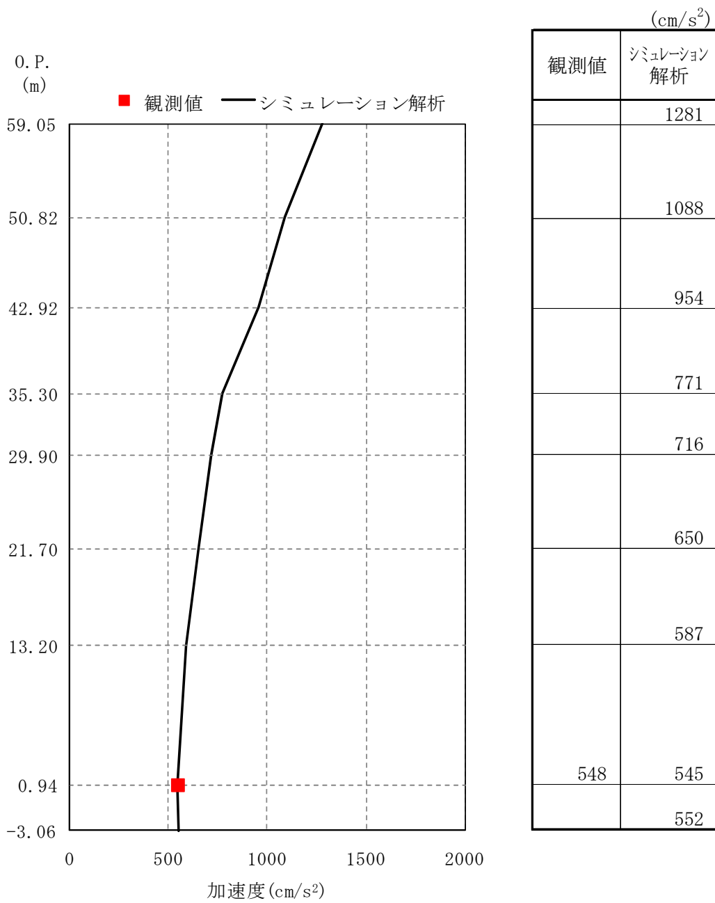
図-3. 5. 1 (2) 最大応答加速度 (東西方向)
