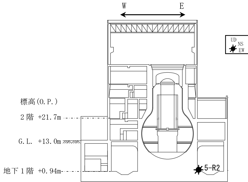
(a) 断面図
