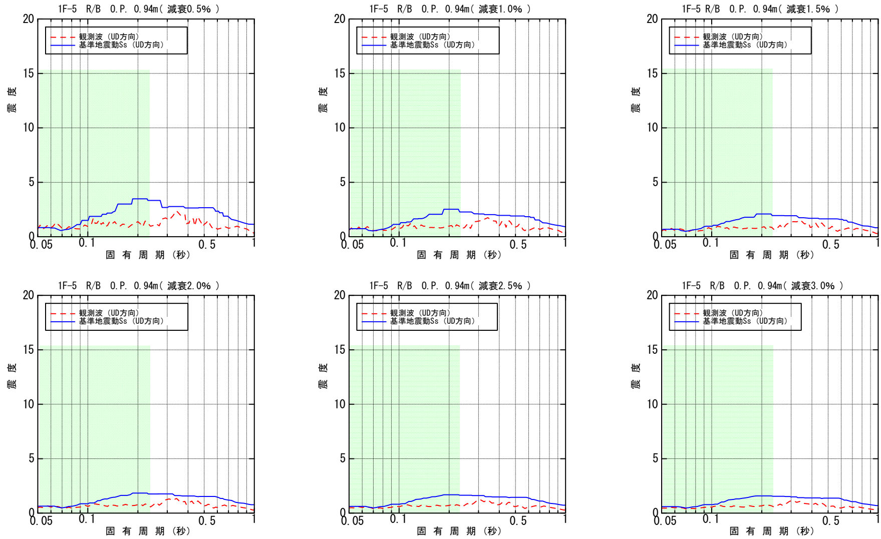
図-4.4.3.6 原子炉建屋 O.P. 0.94m 床応答スペクトル (鉛直方向)
