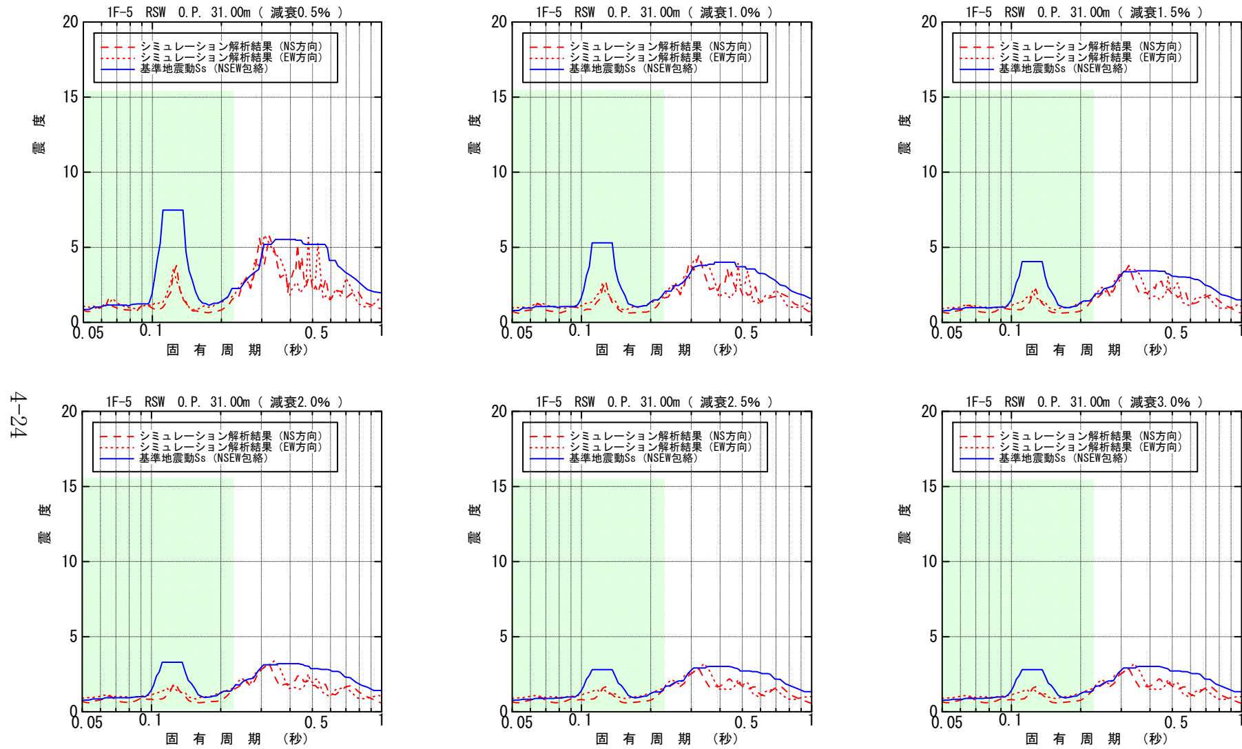
図-4.4.3.7 原子炉遮へい壁 O.P. 31.00m 床応答スペクトル (水平方向)
