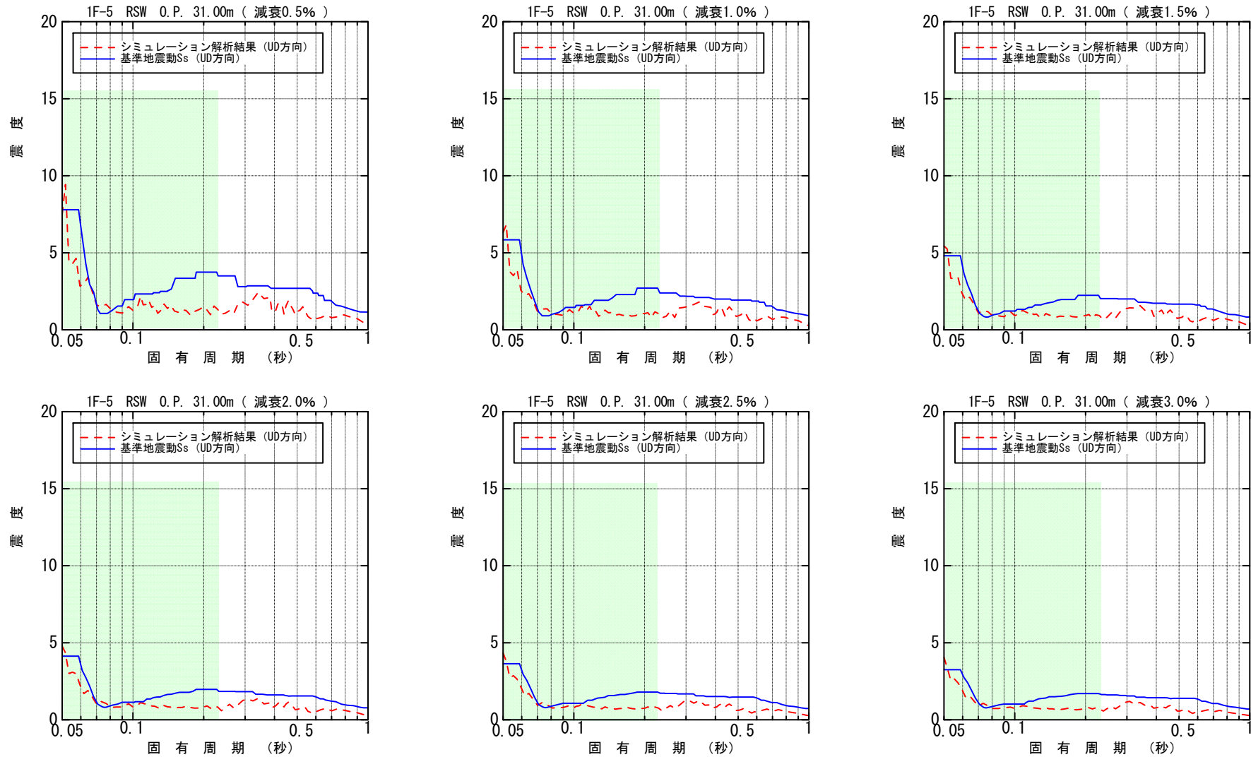
図-4.4.3.10 原子炉遮へい壁 O.P. 31.00m 床応答スペクトル (鉛直方向)
