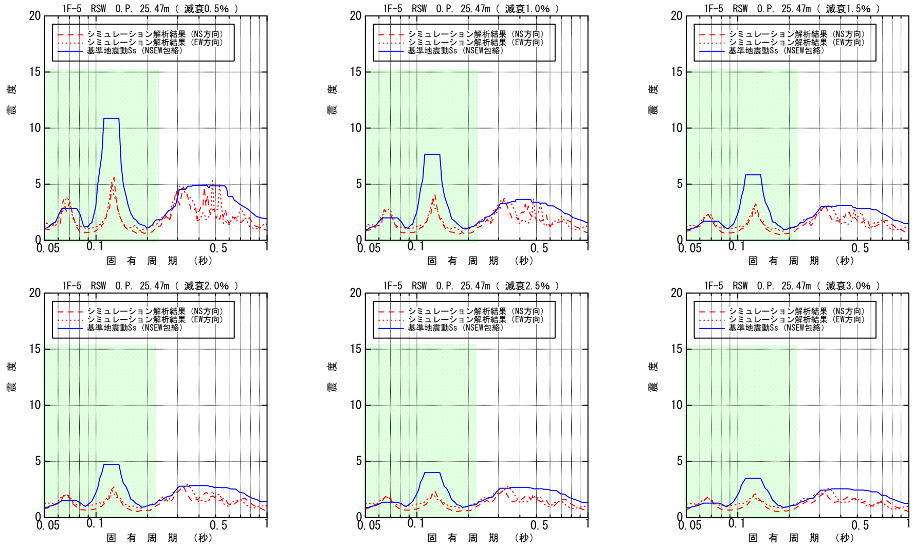
図-4.4.3.8 原子炉遮へい壁 O.P. 25.47m 床応答スペクトル (水平方向)
