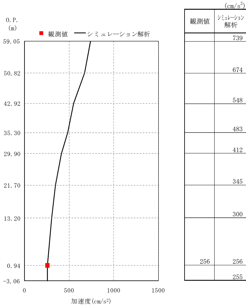
図-3. 5. 1 (3) 最大応答加速度 (鉛直方向)
