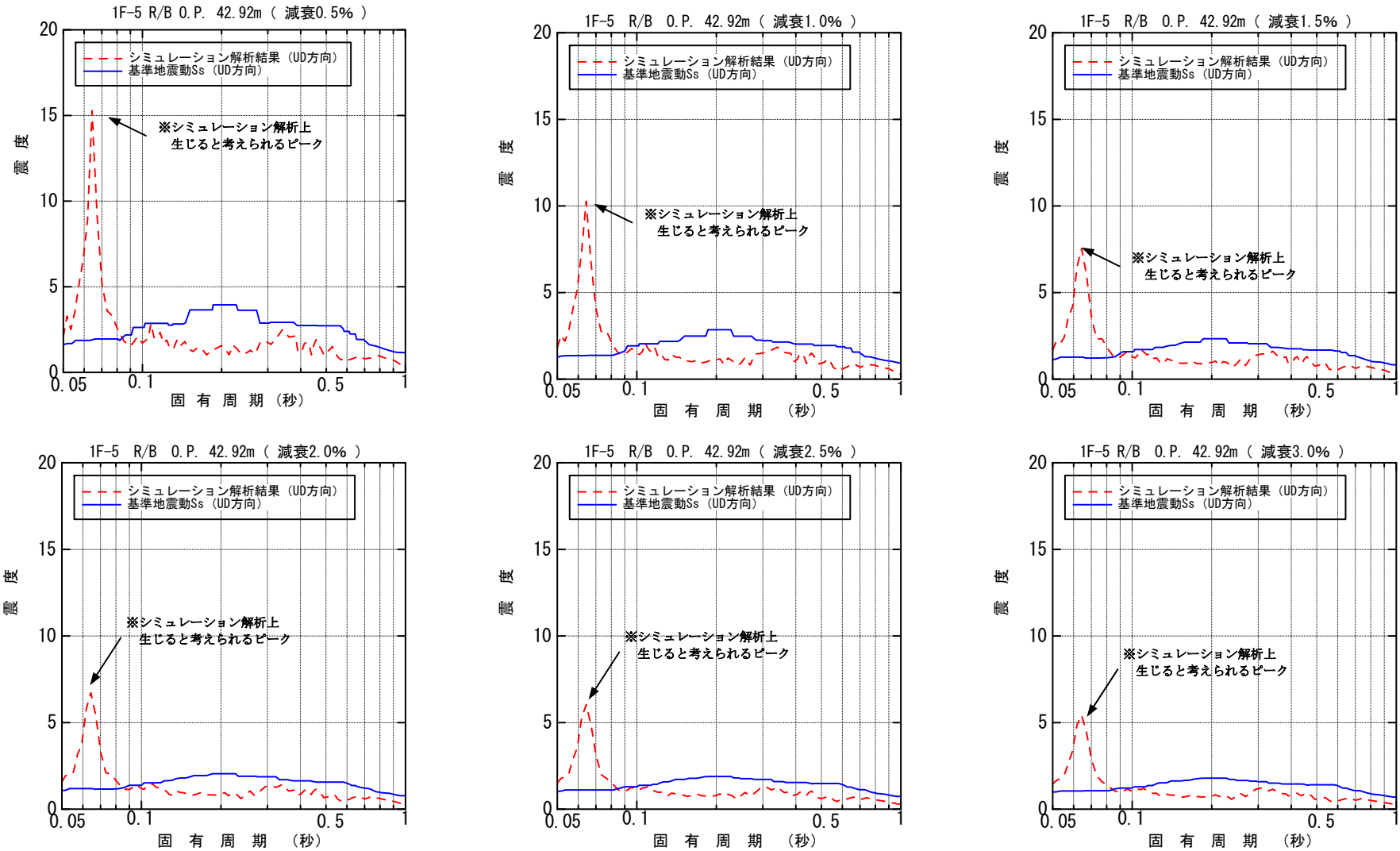
図-4.4.3.4 原子炉建屋 O.P. 42.92m 床応答スペクトル (鉛直方向)
