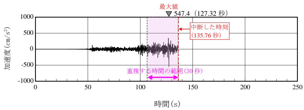
参図-1.2 分類Bの記録 (5-R2 観測点東西方向の例)
