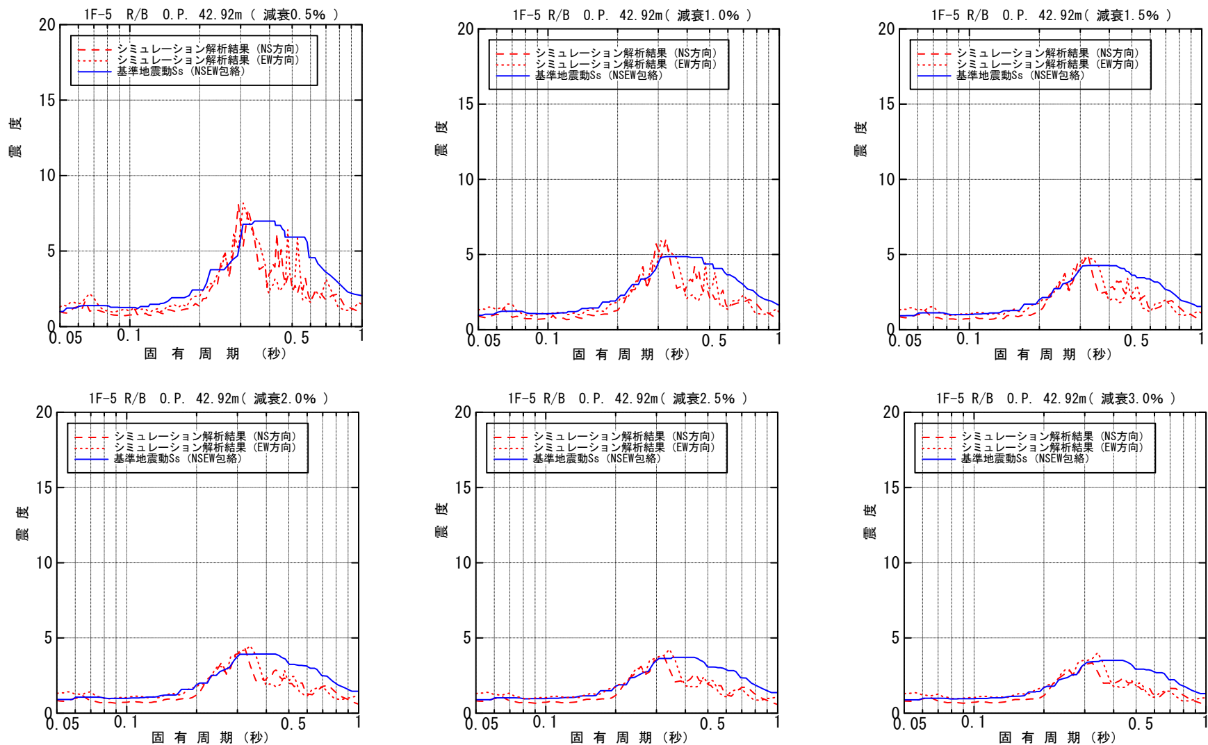
図-4.4.3.1 原子炉建屋 O.P. 42.92m 床応答スペクトル (水平方向)
