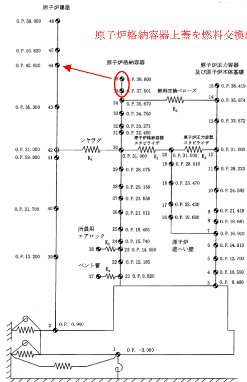
(原子炉建屋—原子炉格納容器—原子炉圧力容器連成系モデル、水平方向) 図-4.4.2.1.1 耐震安全性評価で用いたモデルからの変更 (福島第一5号機)
