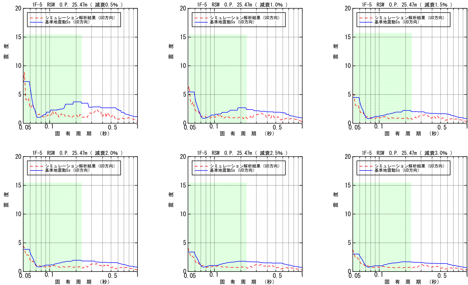
図-4.4.3.11 原子炉遮へい壁 O.P. 25.47m 床応答スペクトル (鉛直方向)
