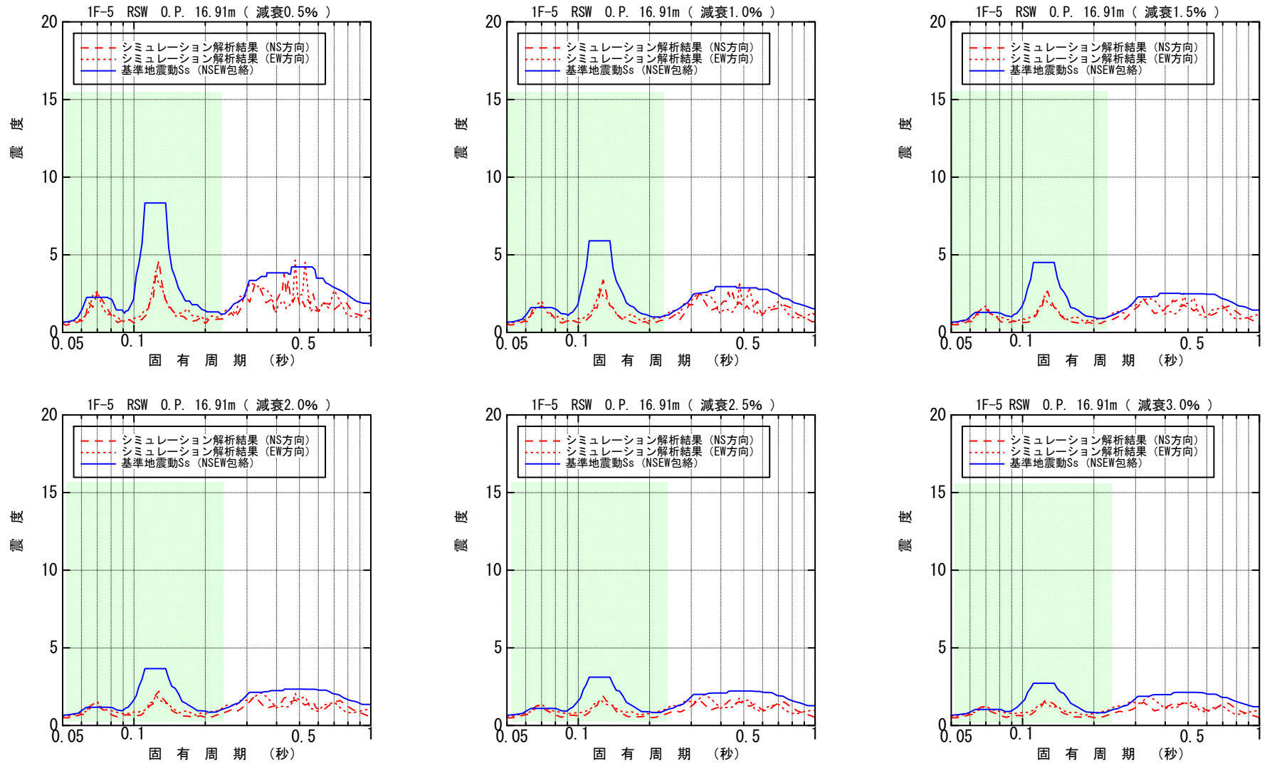
図-4.4.3.9 原子炉遮へい壁 O.P. 16.91m 床応答スペクトル (水平方向)
