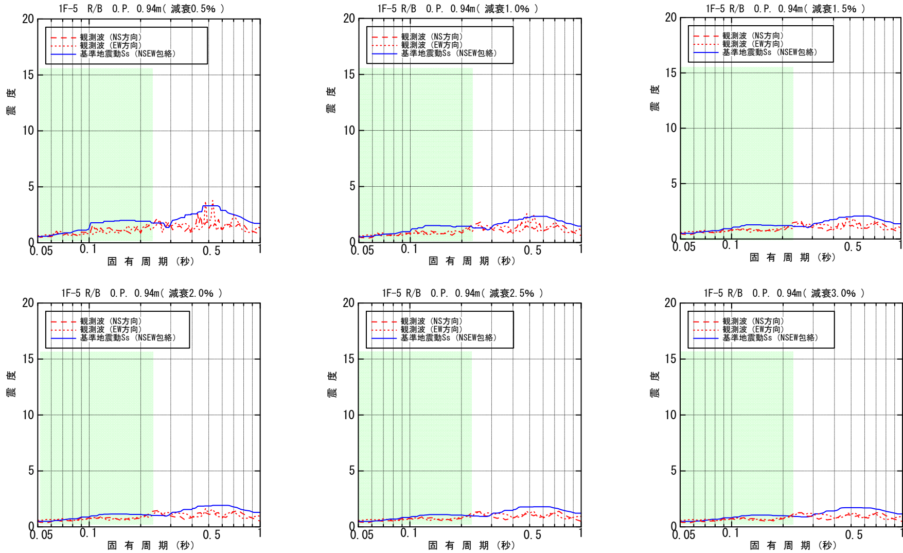
図-4.4.3.3 原子炉建屋 O.P. 0.94m 床応答スペクトル (水平方向)
