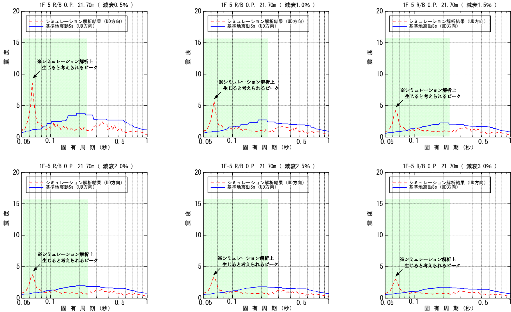
図-4.4.3.5 原子炉建屋 O.P. 21.70m 床応答スペクトル (鉛直方向)
