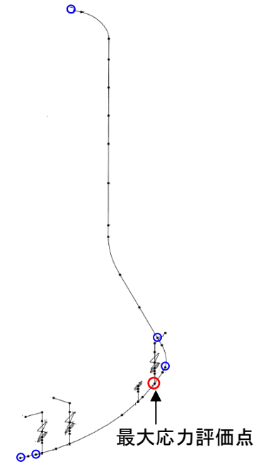
主蒸気系配管モデル (一部)
