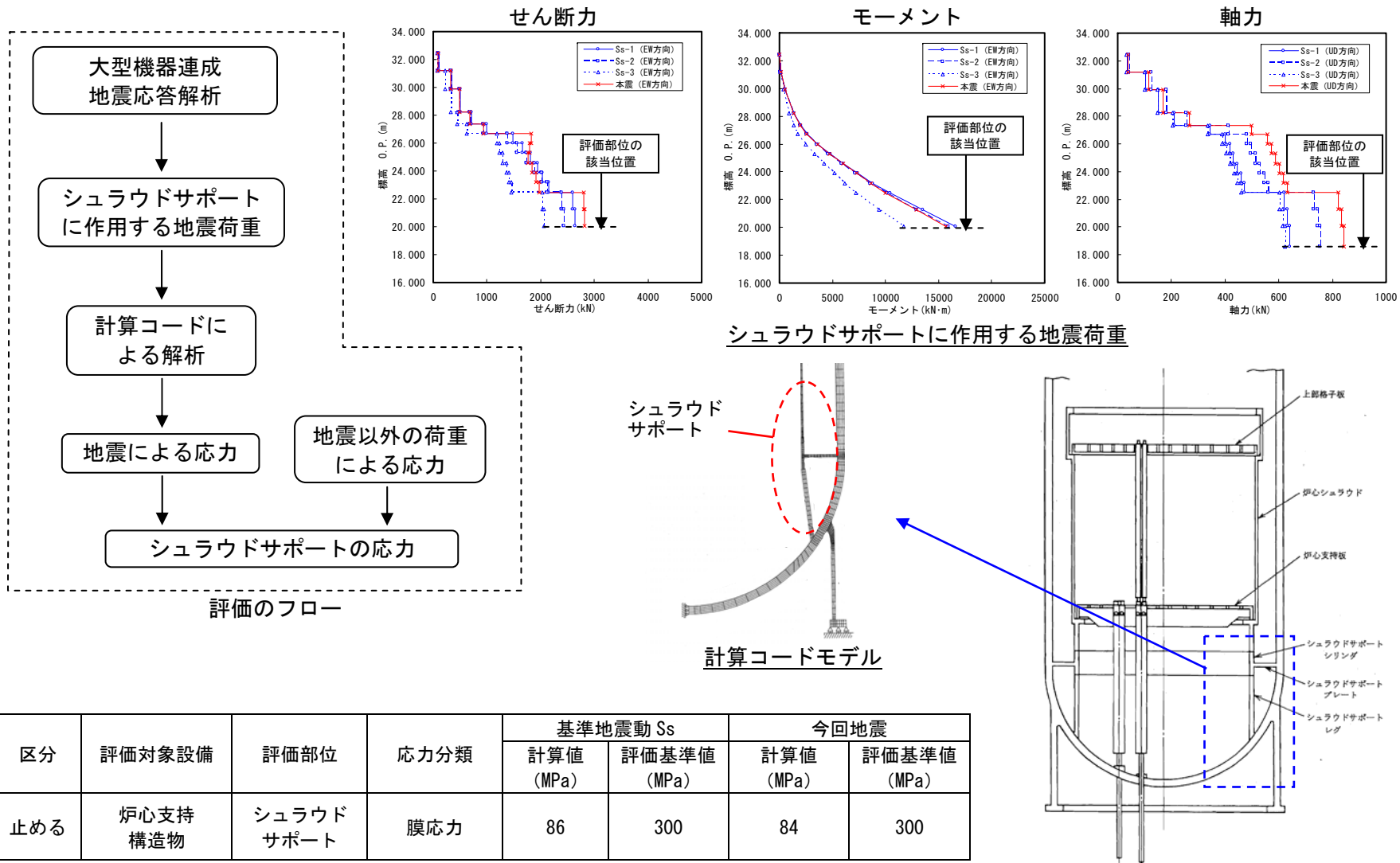
添図-1.1 炉心支持構造物の耐震性評価の概要
