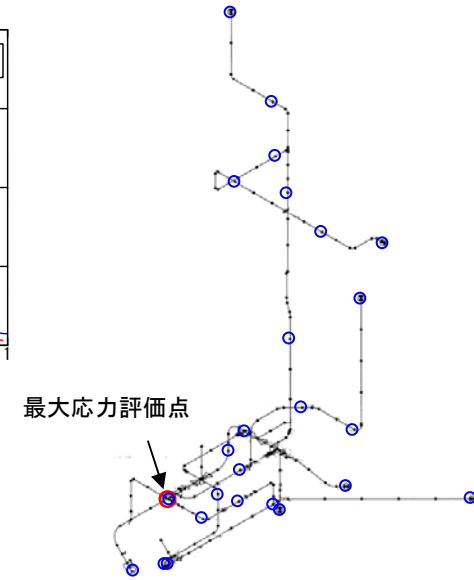
残留熱除去系配管モデル
