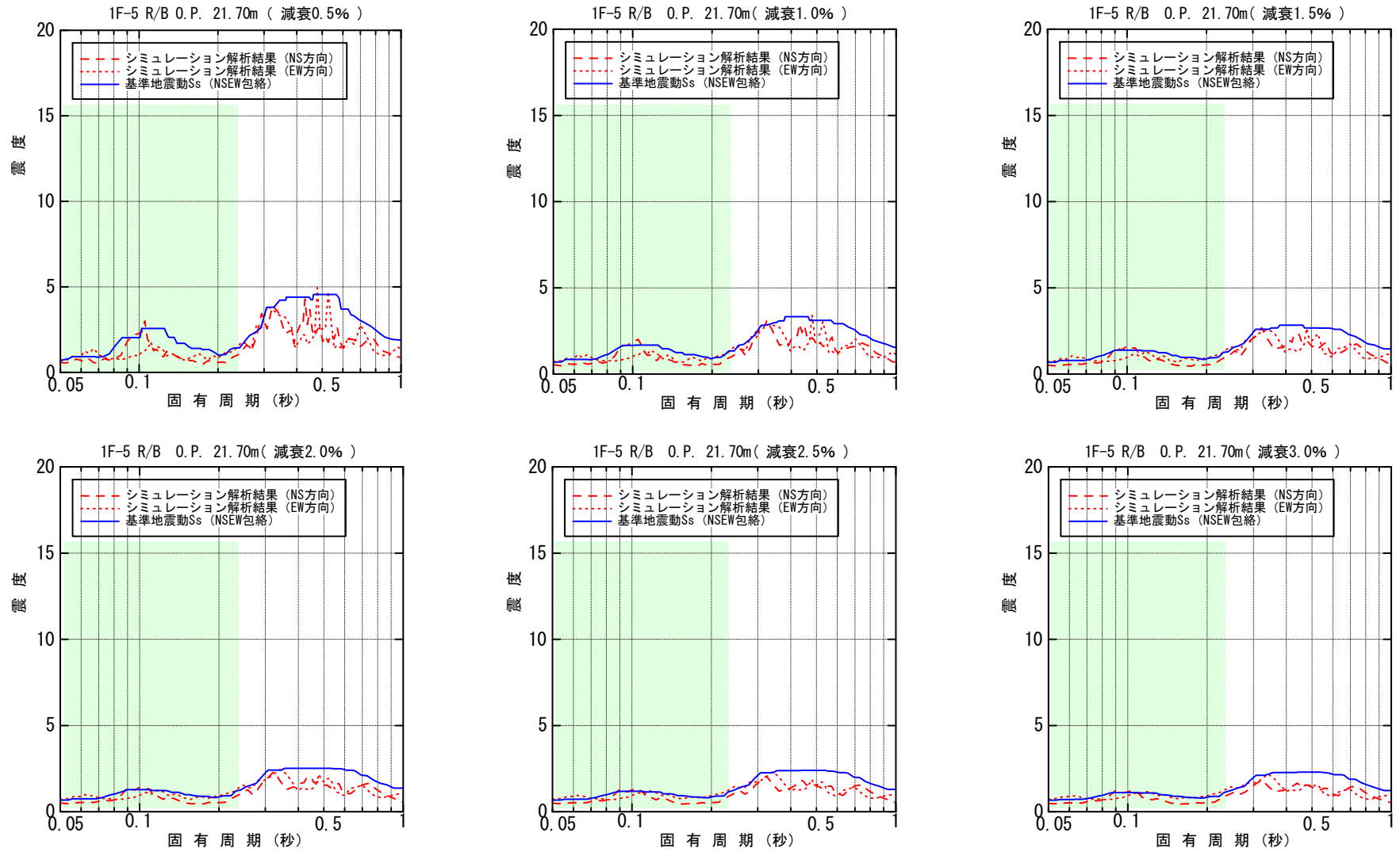
図-4.4.3.2 原子炉建屋 0.P. 21.70m 床応答スペクトル (水平方向)
