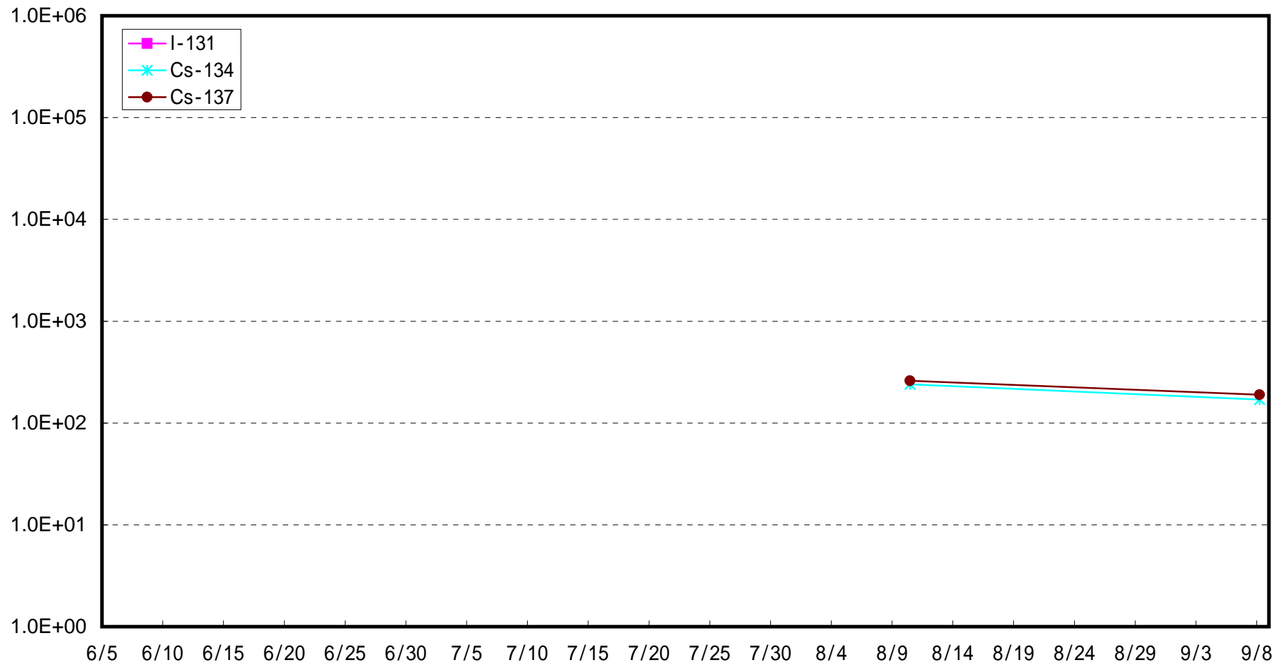
小名浜港沖合3 km海底土放射能濃度 (Bq / kg)
