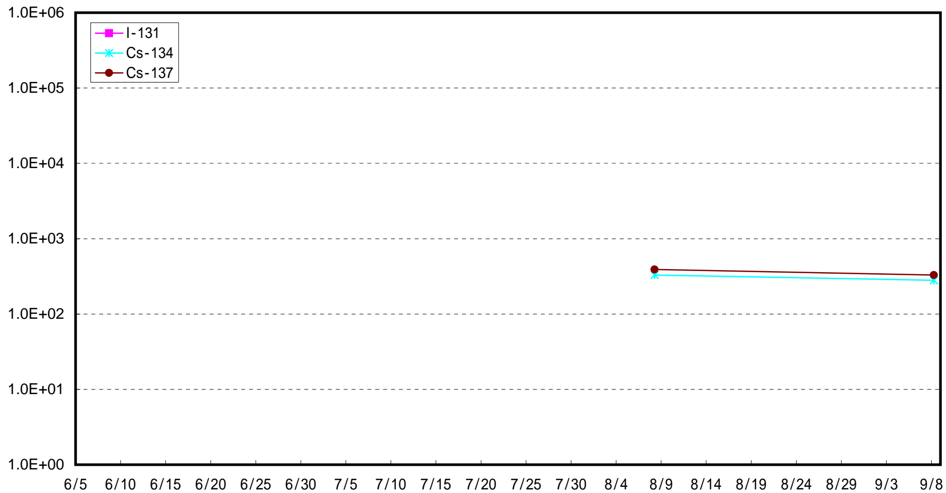
豊間沖合3 km海底土放射能濃度 (Bq / kg)
