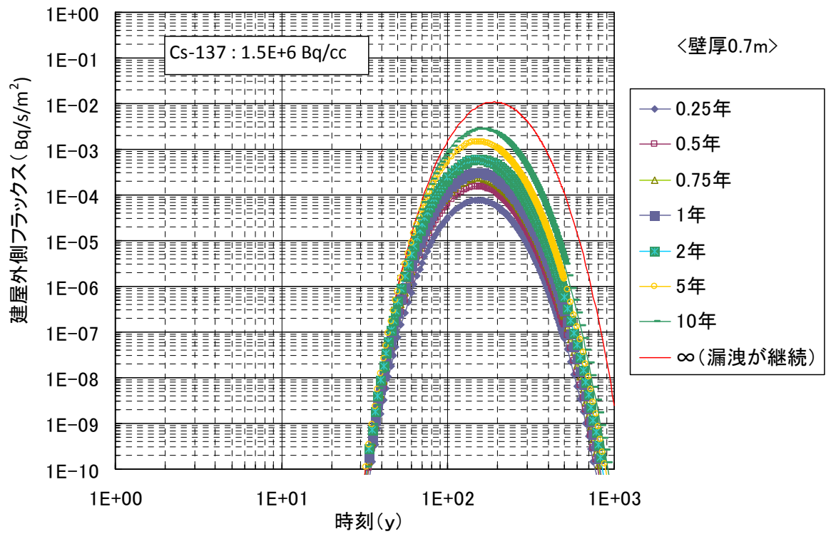
図-2 (2) 建屋からの流出フラックス (側壁 0.7m)
