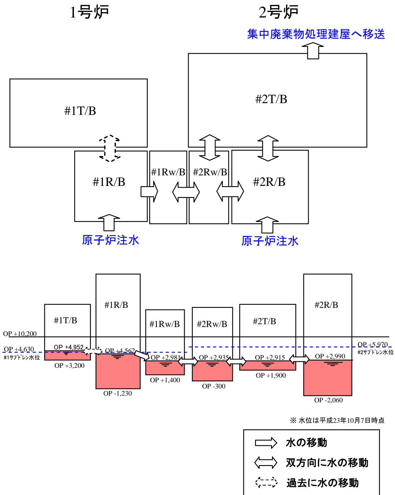
図6-2(1) 1/2号炉建屋間における滞留水の流れのイメージ
