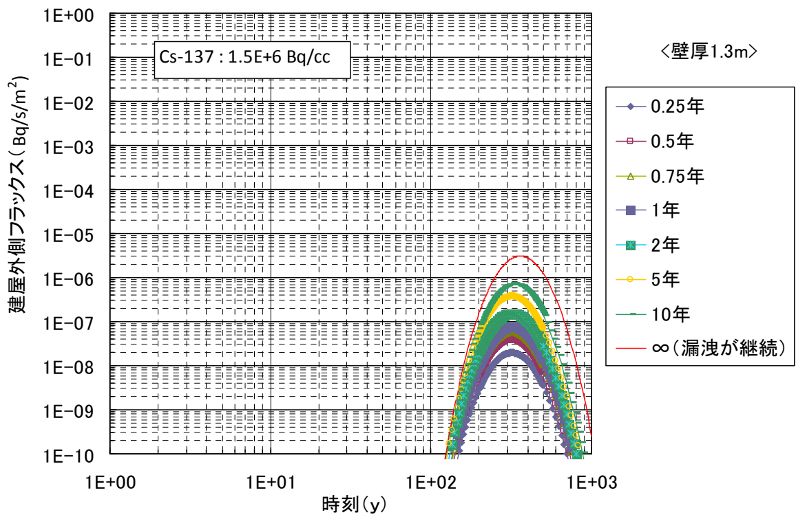
図-2 (4) 建屋からの流出フラックス (側壁 1.3m)
