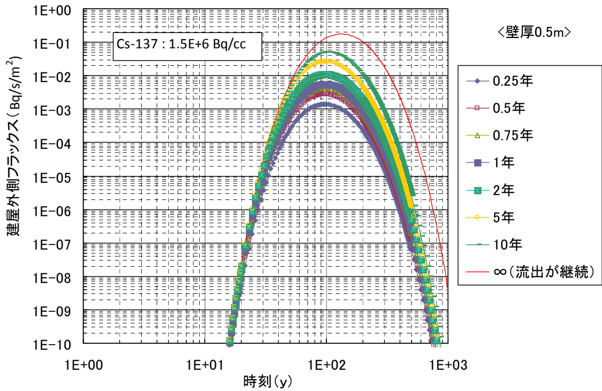
図-2 (1) 建屋からの流出フラックス (側壁 0.5m)
