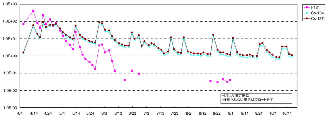
①1号炉サブドレン水放射能濃度 (Bq/cm 3 )
