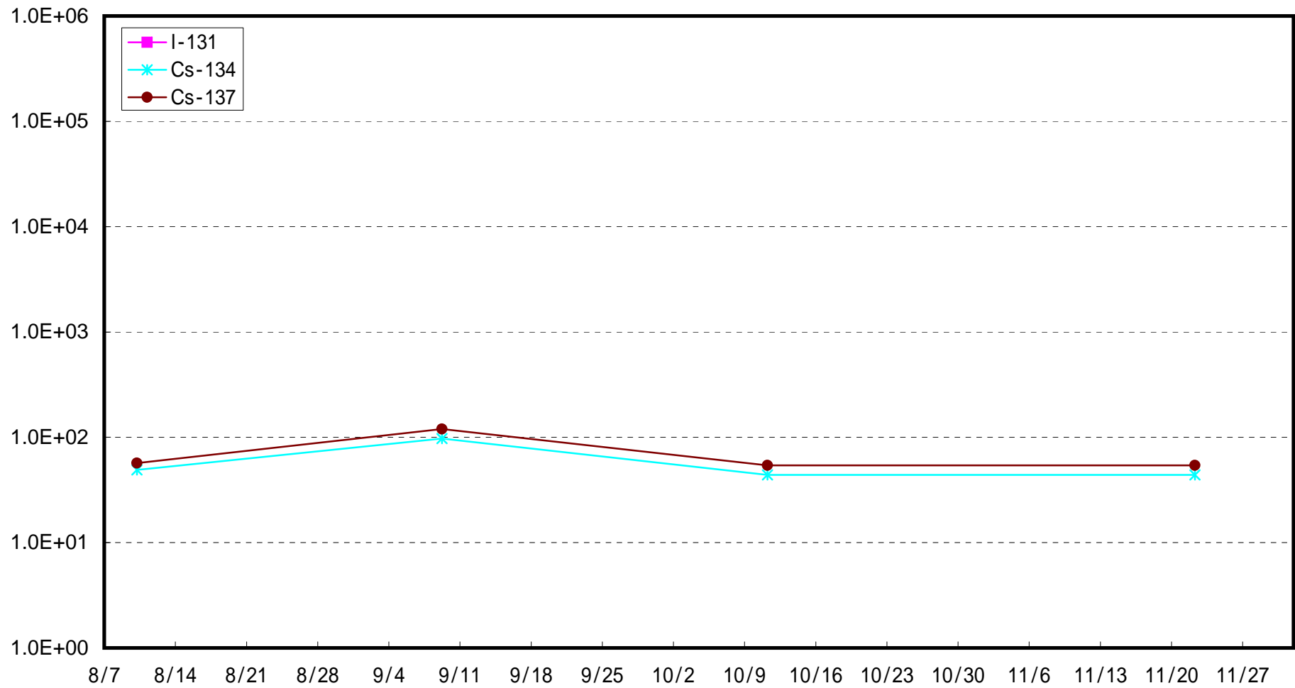
鹿島沖合5 km海底土放射能濃度 (Bq / kg · 湿土)
