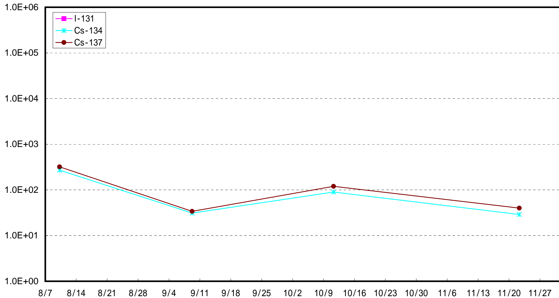
相馬市沖合5 km海底土放射能濃度 (Bq / kg·湿土)
