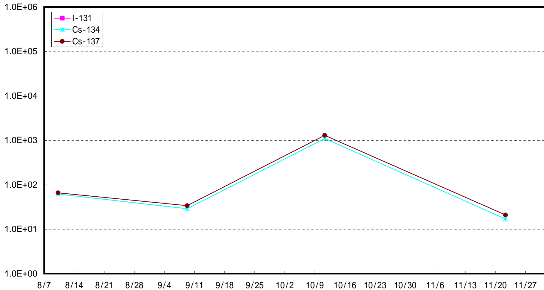
相馬市沖合3 km海底土放射能濃度 (Bq / kg·湿土)
