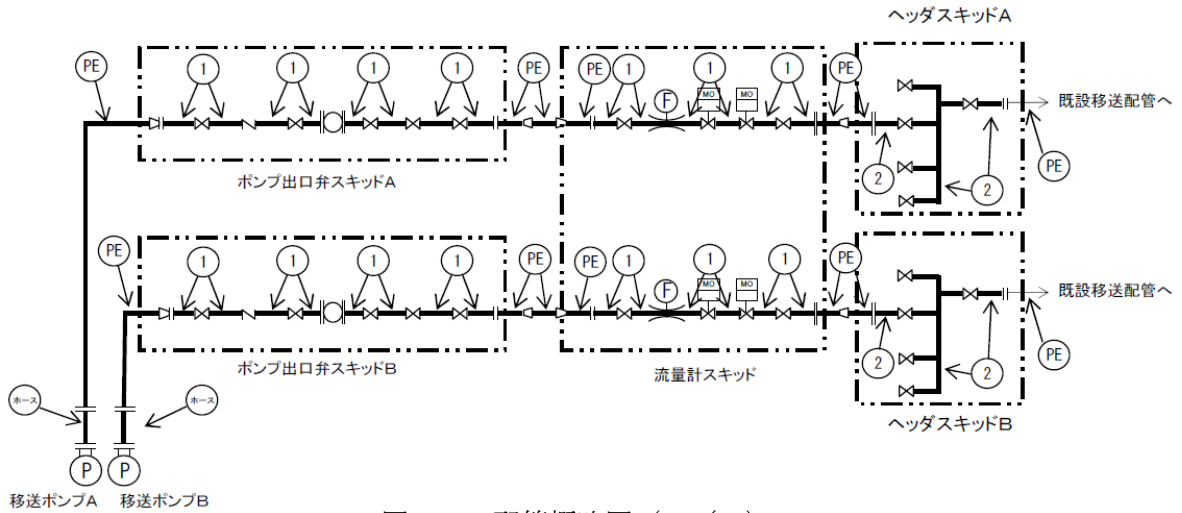
図-1 配管概略図（1 / 2）
