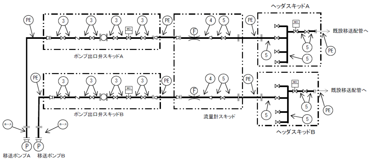
図-1 配管概略図（2 / 2）
