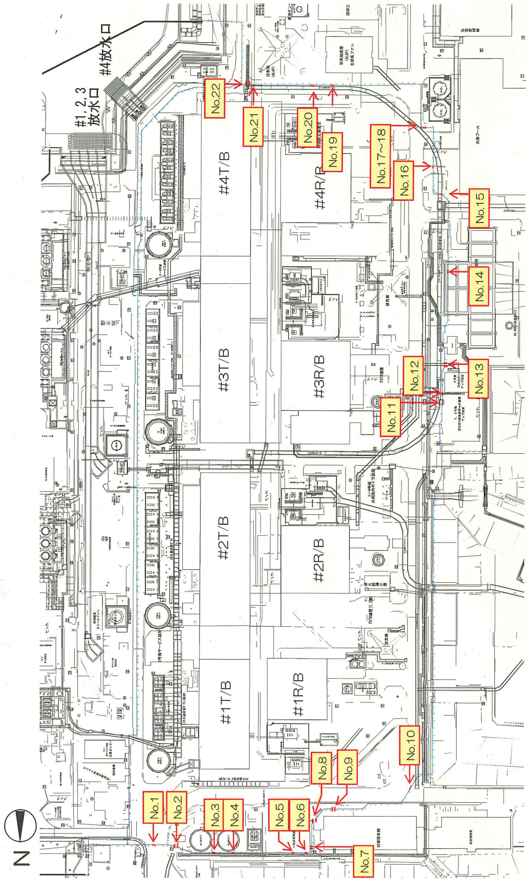
図1 試験凍結箇所
