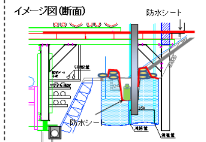
削孔箇所地上部漏えい対策例2
