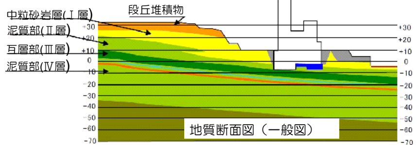
図1 1～4号機建屋周辺の地層構成
