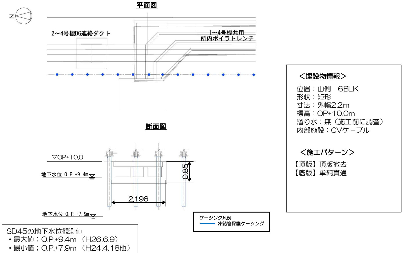
図 1 6 - 1 3 【 6 - 4 】 1 ~ 4 号機共用所内ボイラートレンチ 施工方法（貫通施工）
