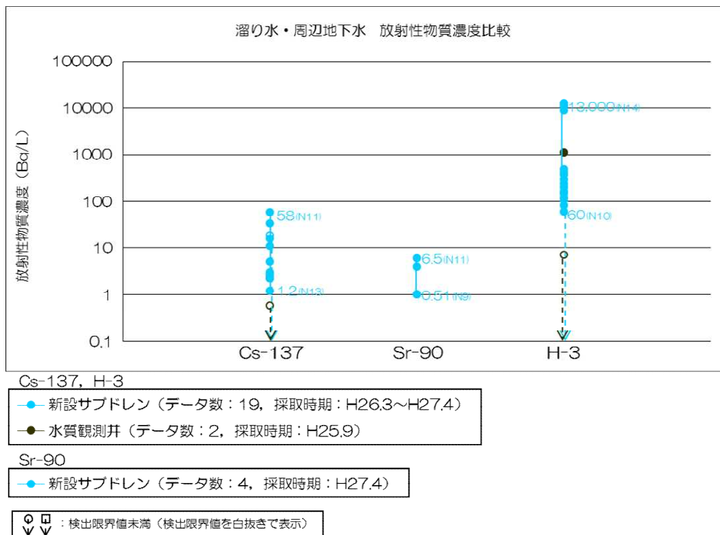
図 1 5 埋設物内に溜り水を有する貫通箇所周辺の地下水 (サブドレンピット・観測井) の放射性物質濃度分布
