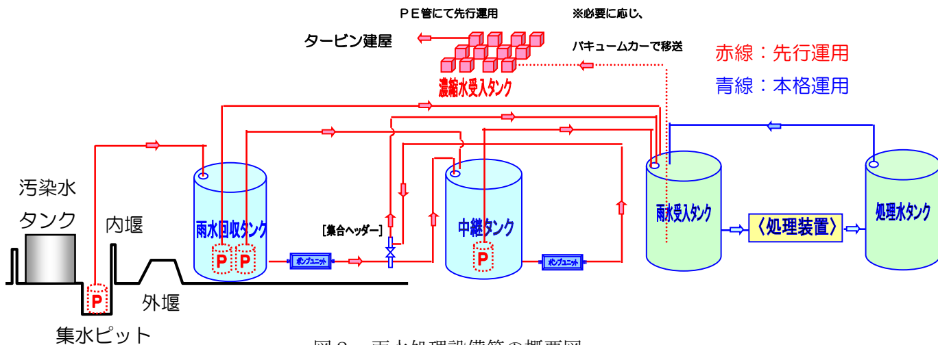
図2 雨水処理設備等の概要図
