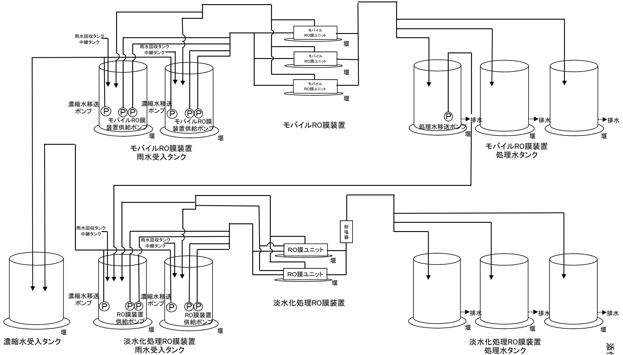
全体概略図 (1/2)
