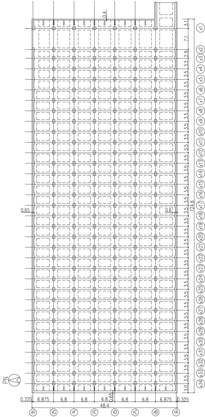
图一 2 地下 2 階平面图 (G. L. -8.7) (单位 : m)
