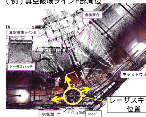
トラス室レーザスキャン点群データ (例)真空破壊ラインE部周辺
