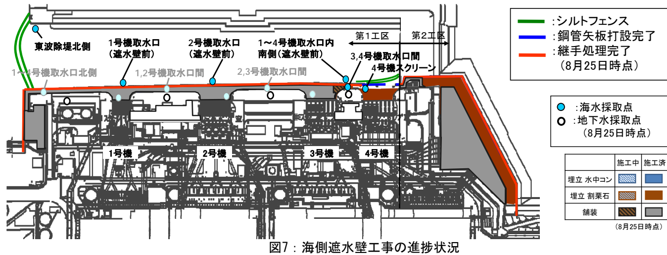
図7：海側遮水壁工事の進捗状況
