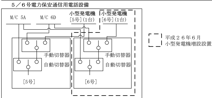
図-1 ページング・電力保安通信用電話設備 電源系統図
