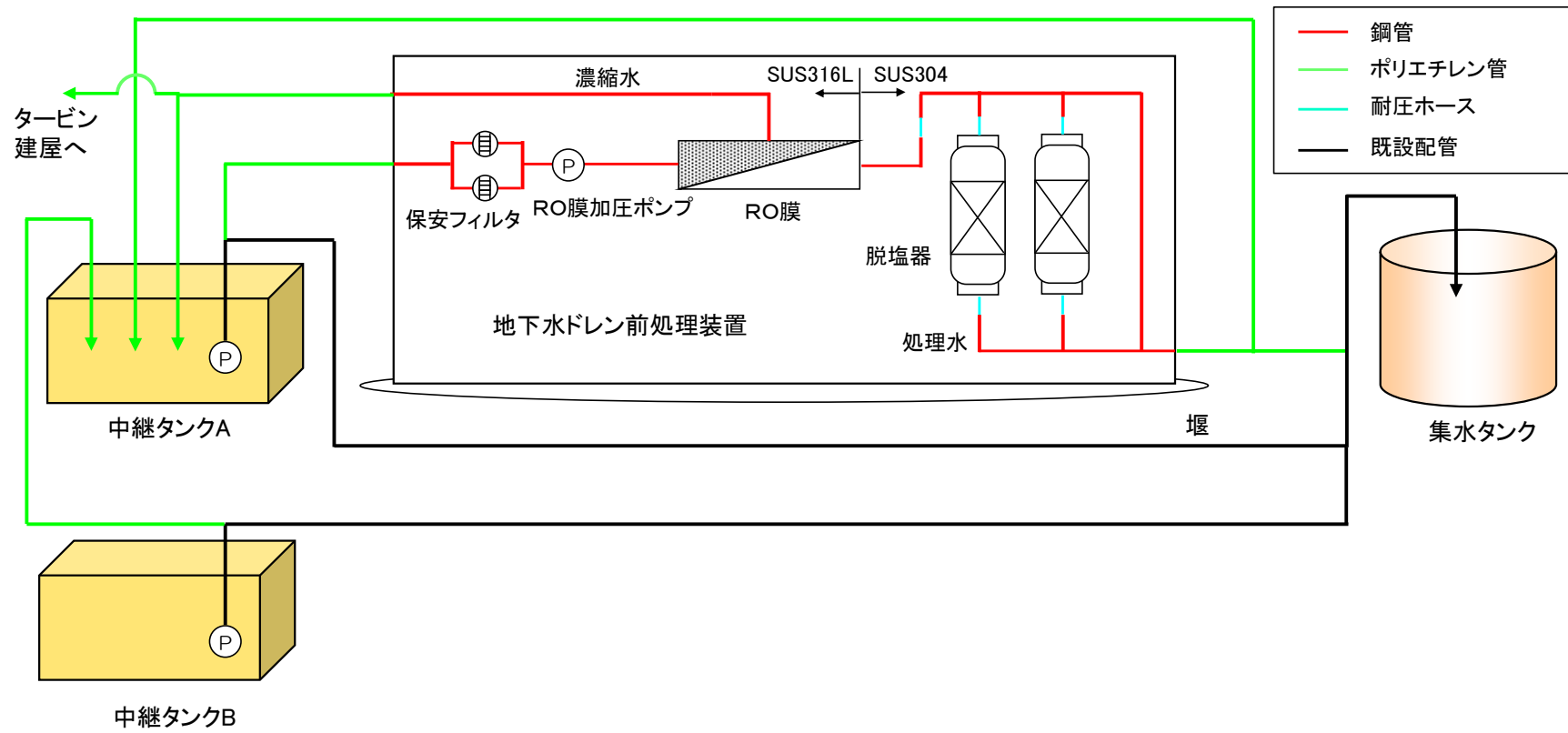
図ー 1 : 地下水ドレン前処理装置及びその周辺機器の全体概略図
