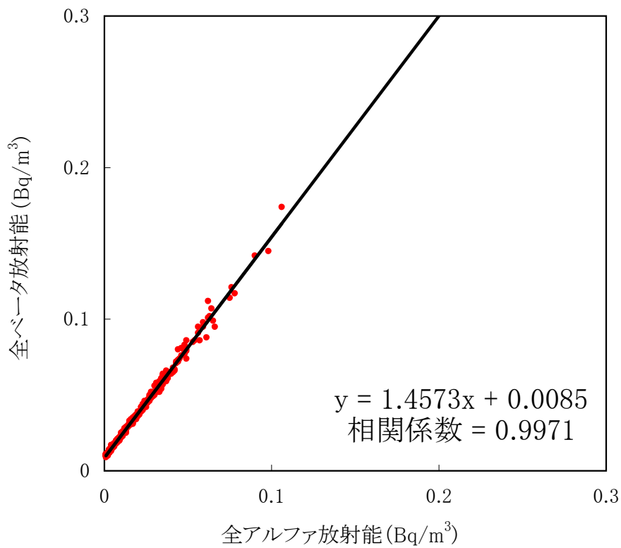
大気浮遊じんの全アルファ・全ベータ放射能の相関図 (MP-1) (平成26年7月～9月)
