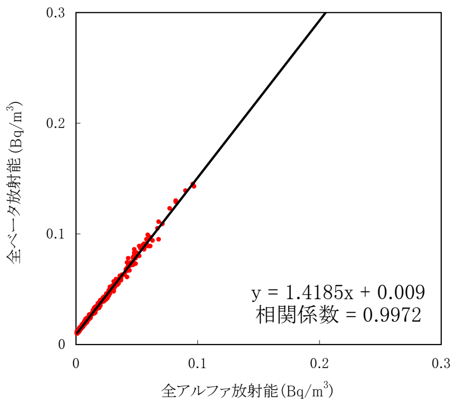
大気浮遊じんの全アルファ・全ベータ放射能の相関図 (MP-7) (平成26年7月～9月)
