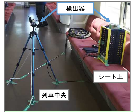
列車内計測器の設置状況
