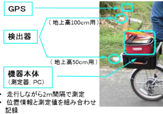
【自転車モニタリング装置の概要】
