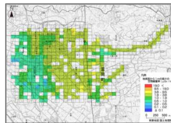
【富岡町の測定結果(100mメッシュ化)※】
