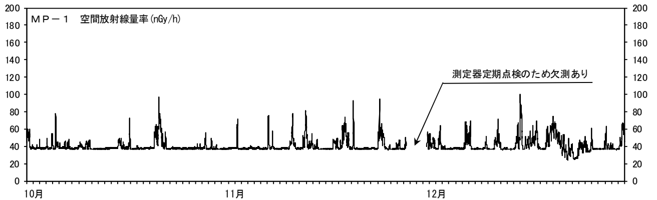
図1 MP-1～3の空間放射線量率と降水量及び積雪深との関係 (測定期間：令和5年10月1日～令和5年12月31日)
