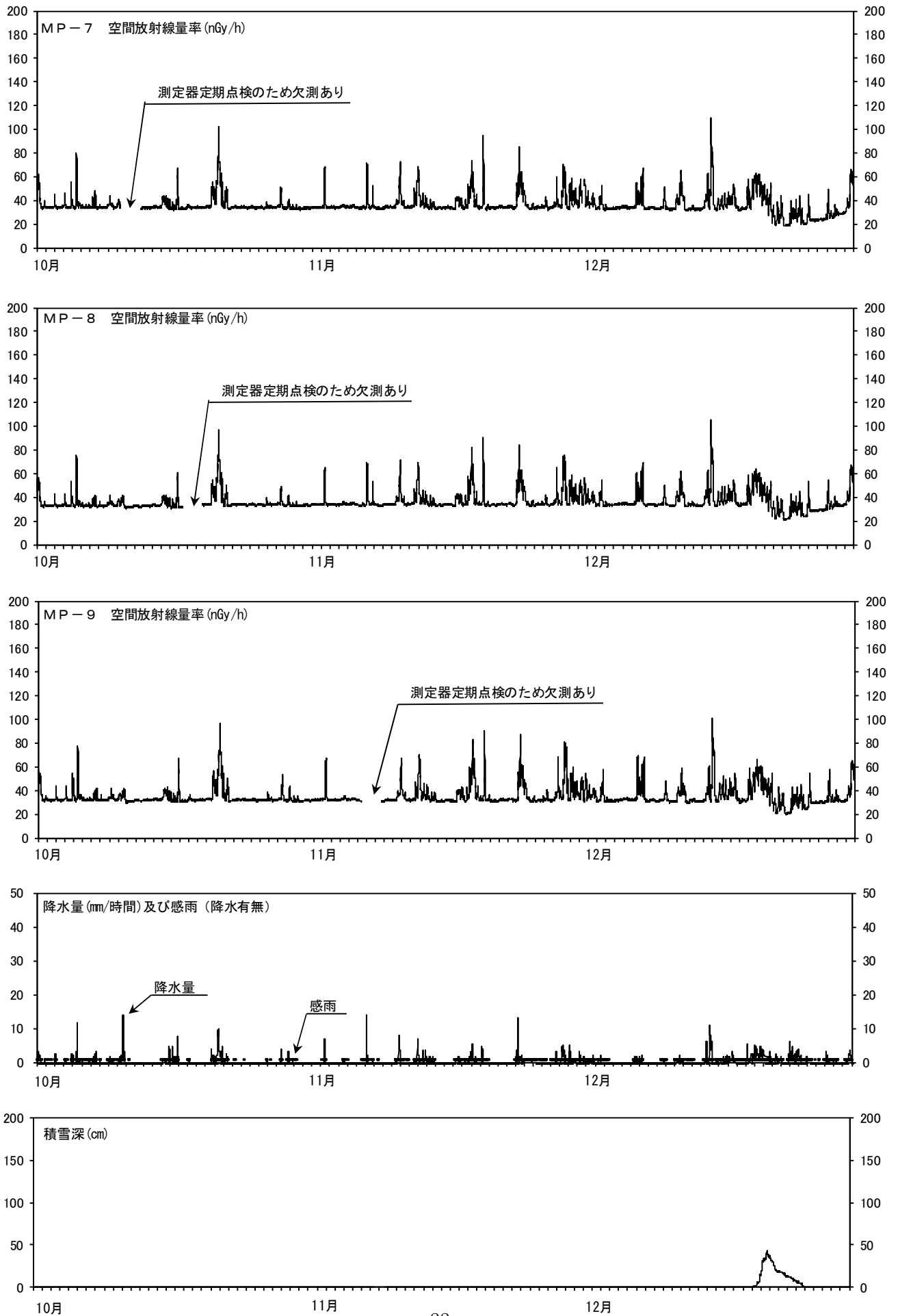
図3 MP-7～9の空間放射線量率と降水量及び積雪深との関係 (測定期間：令和5年10月1日～令和5年12月31日)
