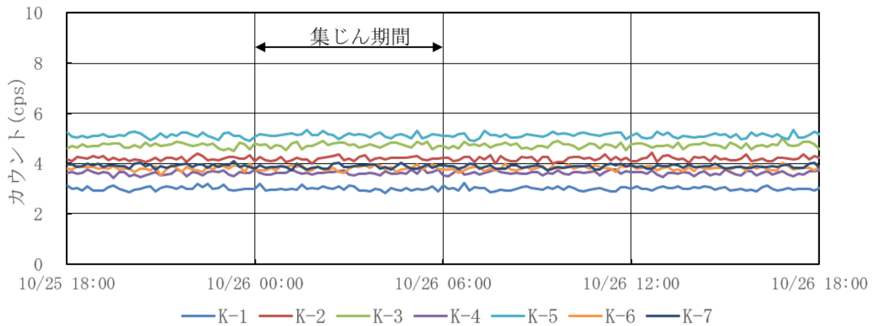
図6 排気筒モニタ指示値の推移 (令和5年10月25日～10月26日)
