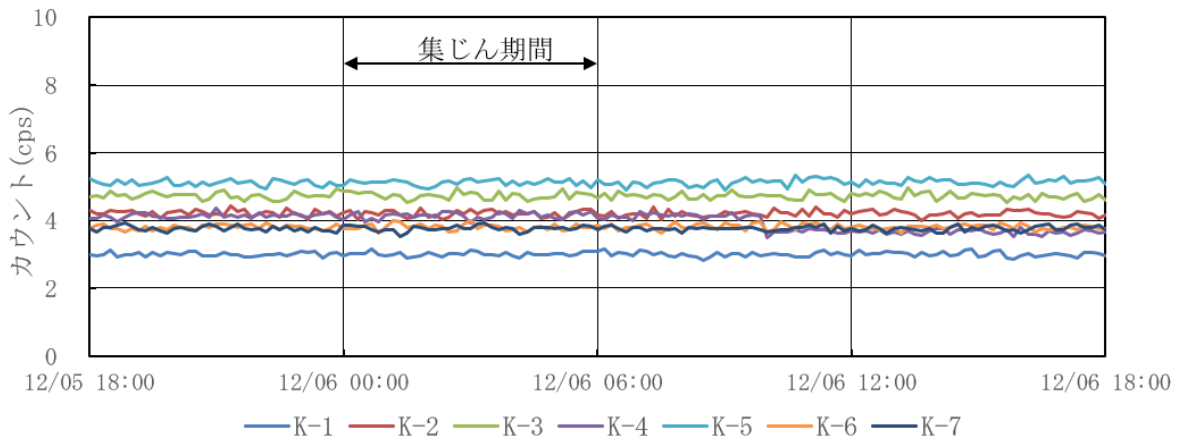
図3 排気筒モニタ指示値の推移 (令和5年12月5日～12月6日)
