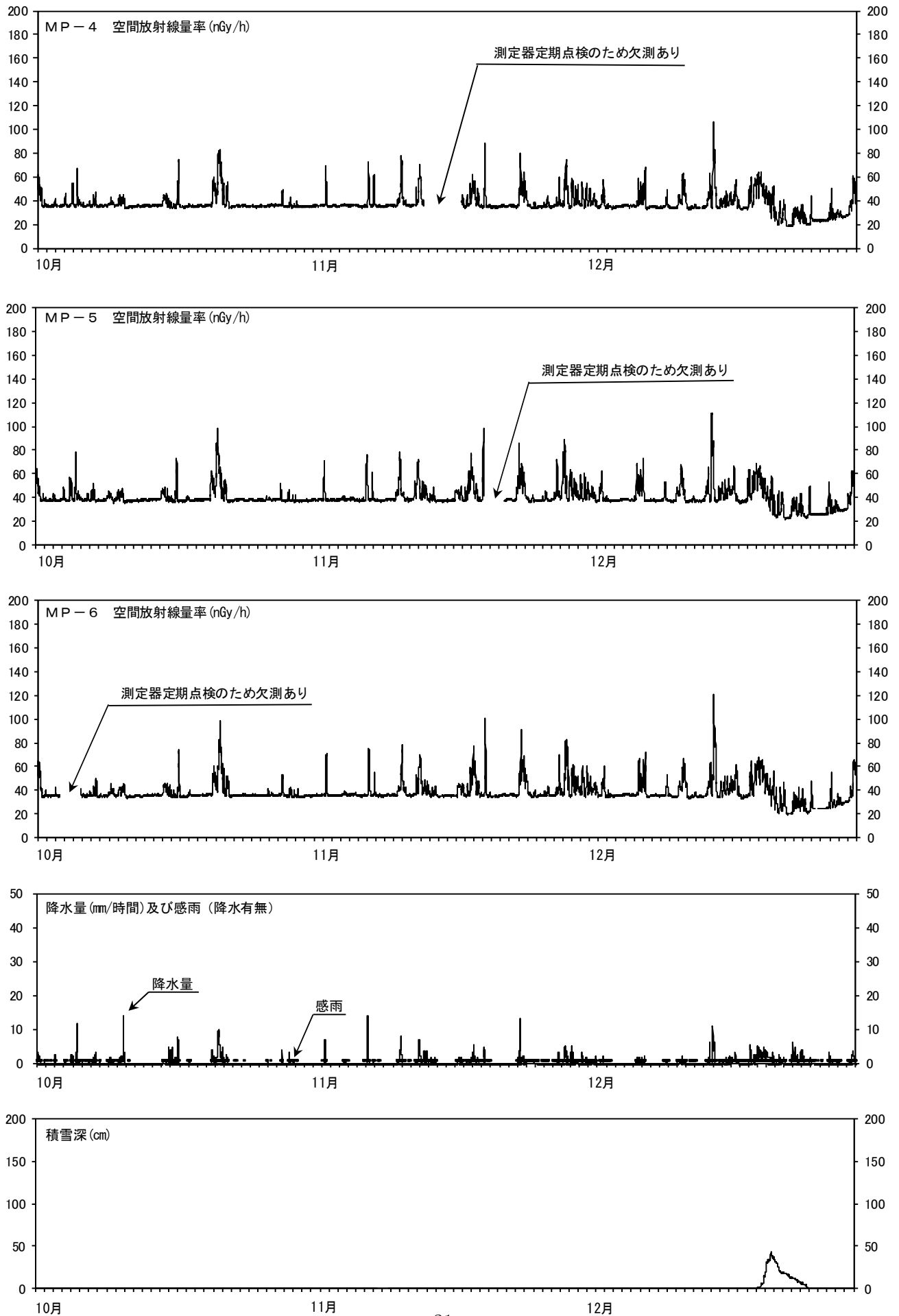
図2 MP-4～6の空間放射線量率と降水量及び積雪深との関係 (測定期間：令和5年10月1日～令和5年12月31日)
