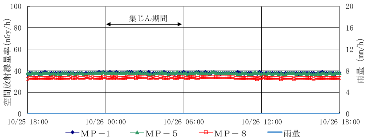
図5 空間放射線量率の推移 (令和5年10月25日～10月26日)
