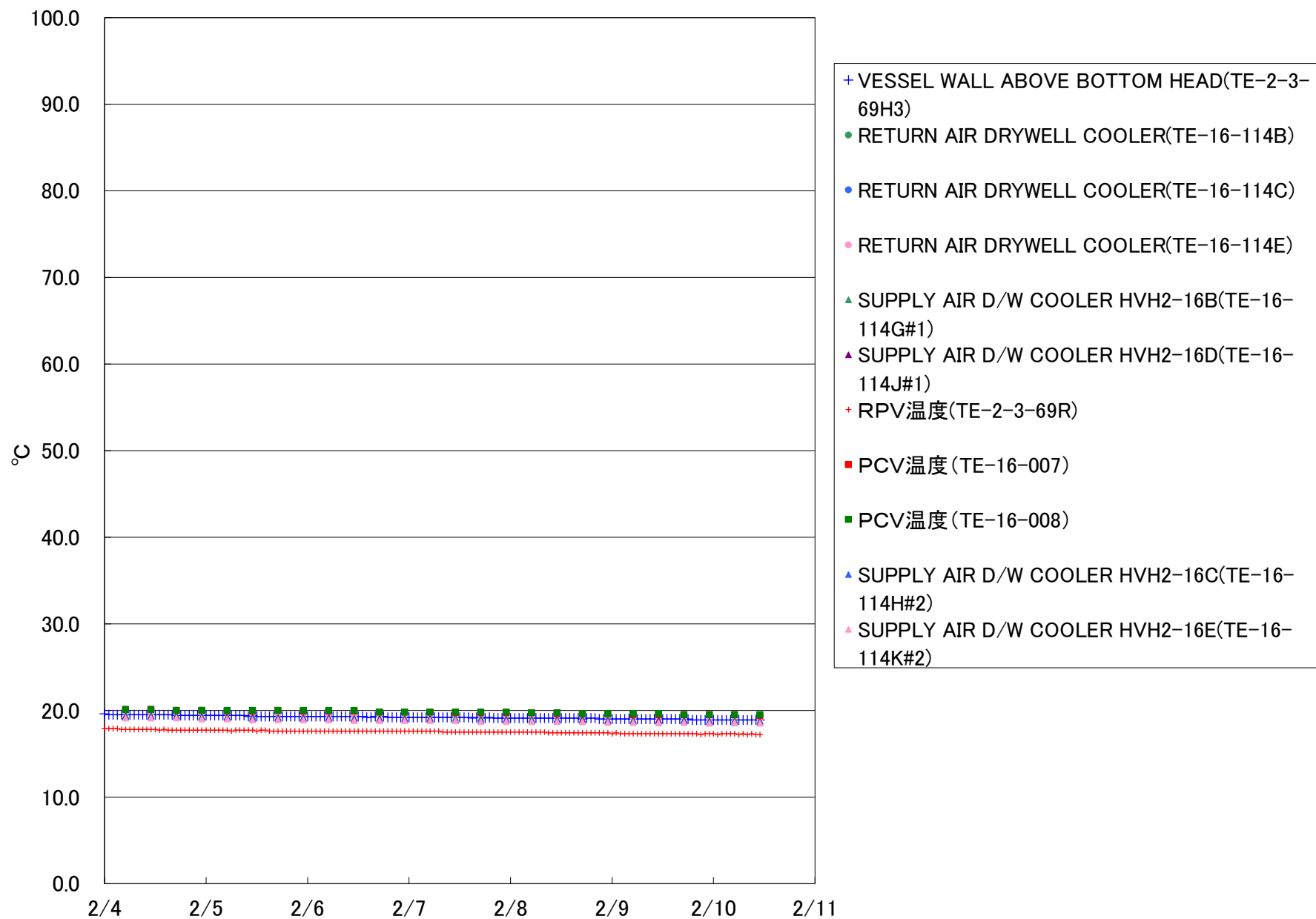
福島第一原子力発電所2号機 温度に関するパラメータ
