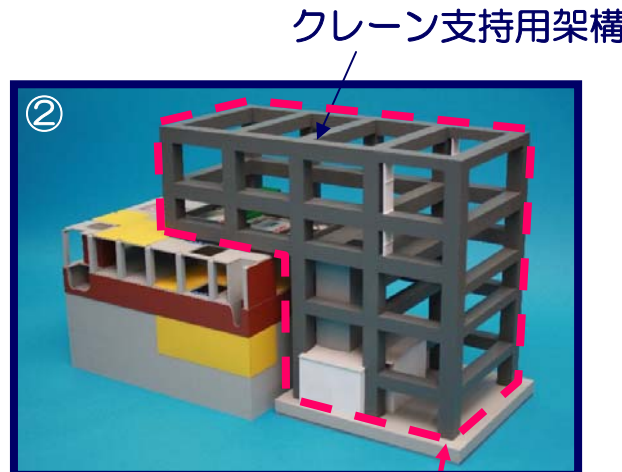
燃料取り出し用カバーの鉄骨設置
