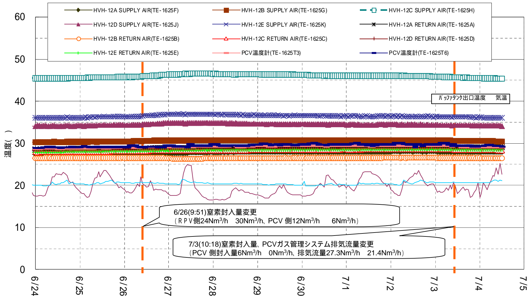
1号機原子炉格納容器内温度グラフ
