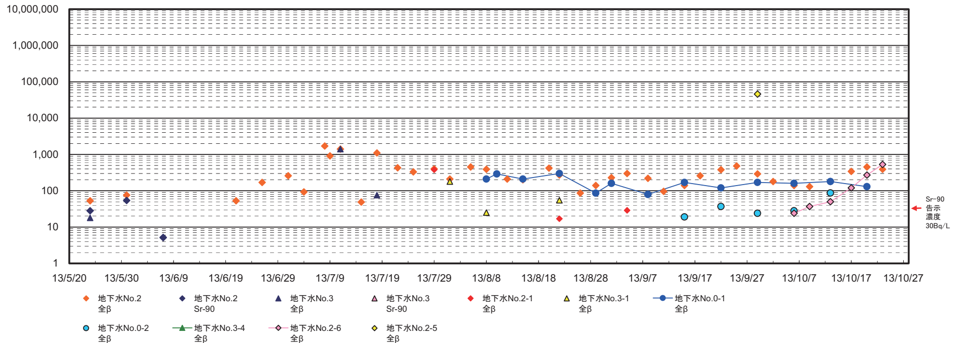
Bq/L 1号機北側、2,3号機取水口間、3,4号機取水口間地下水の全ベータ、ストロンチウム濃度の推移
