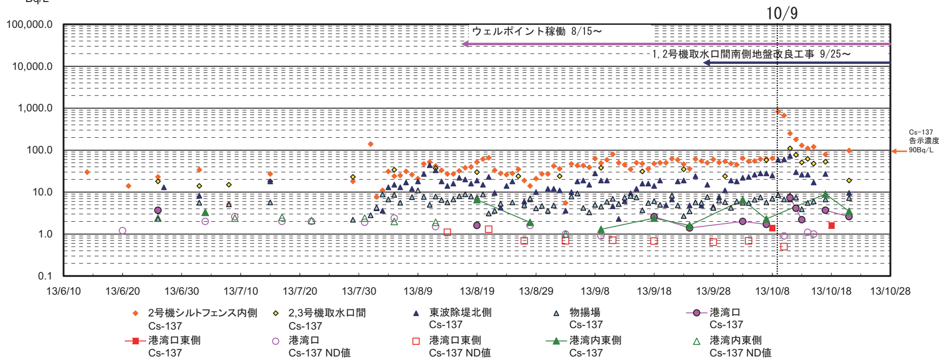
2号機シルトフェンス内側～港湾口東側の海水の濃度推移(Cs-137)
