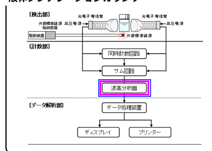
液体シンチレーションカウンター
