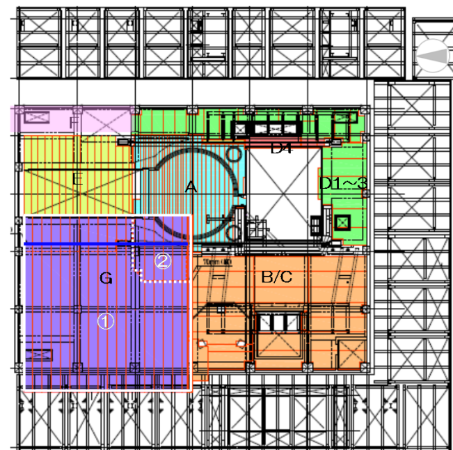
オペレーティングフロア上の遮蔽体設置計画における各工区
