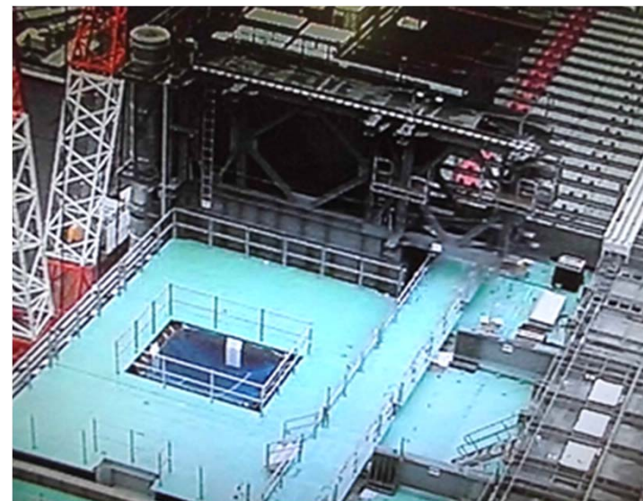
FHMガーダ鉄骨部材 吊り下ろし完了
