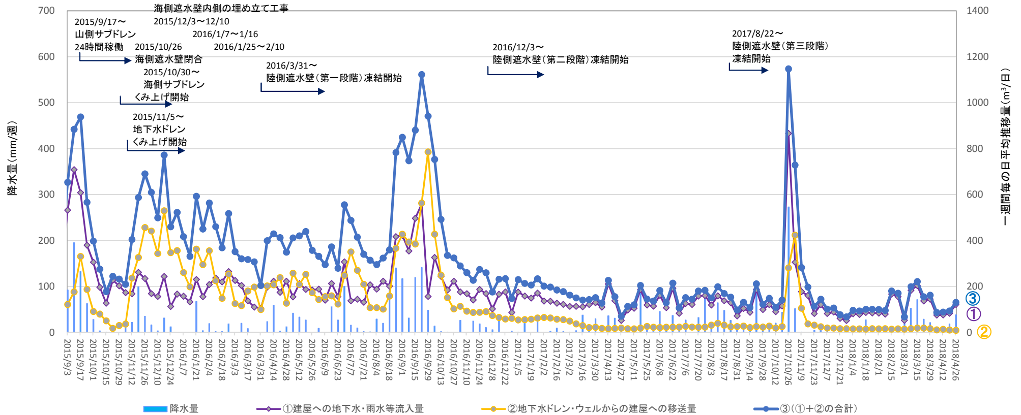
地下水ドレンからタービン建屋への移送量 (2018年4月19日 ~ 2018年4月25日)
