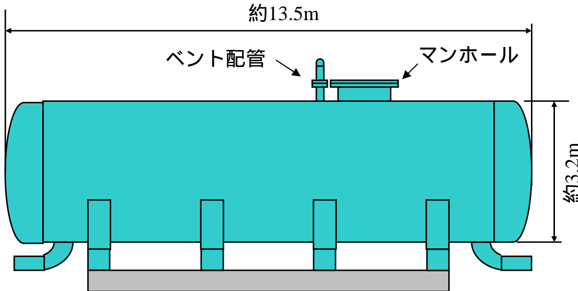
<タンク外観>
