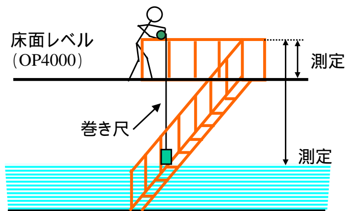
水位測定
