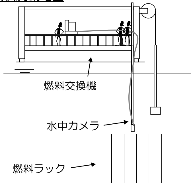
点検状況概略図
