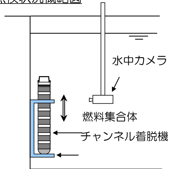
点検状況概略図
