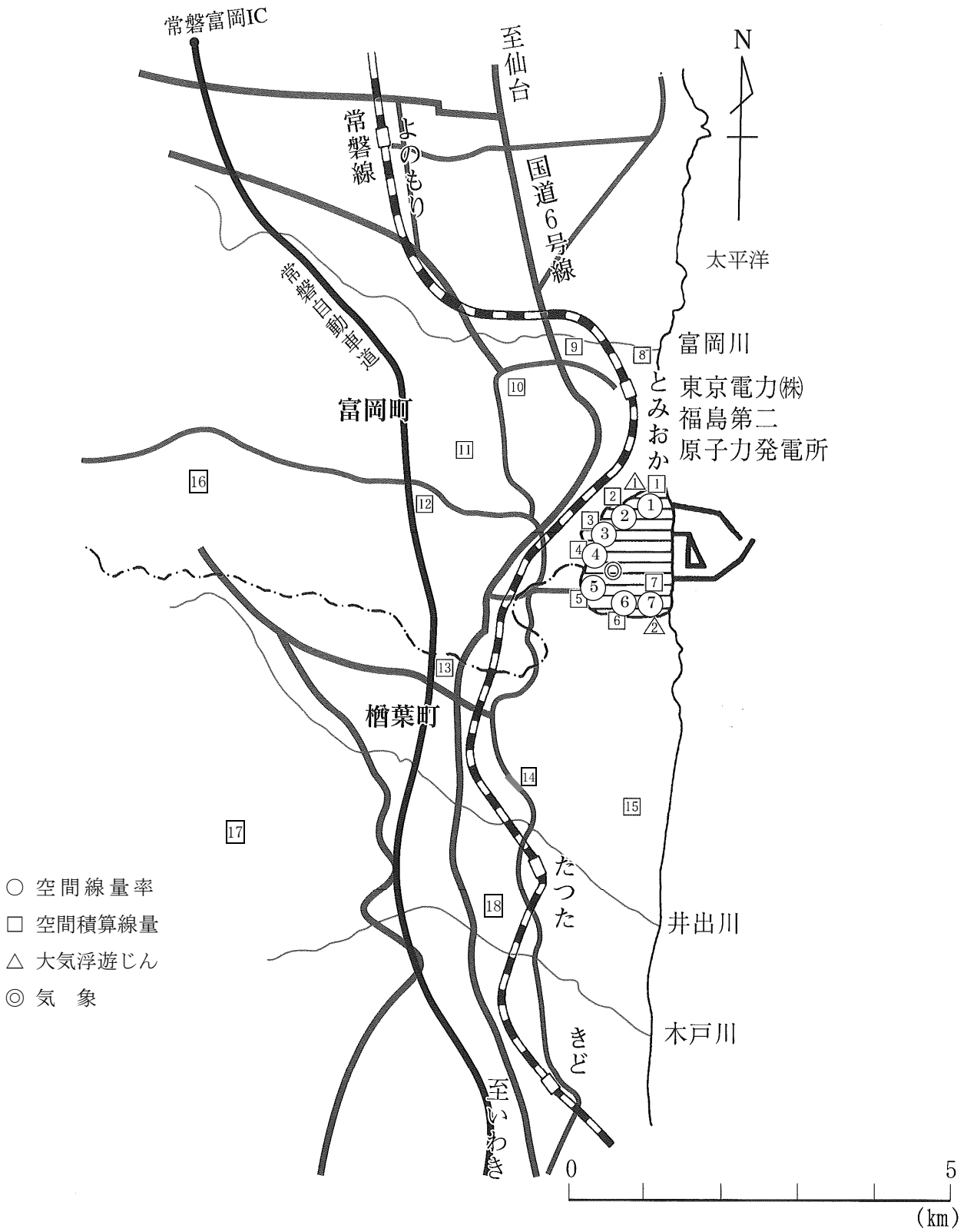
図-1 測定地点
