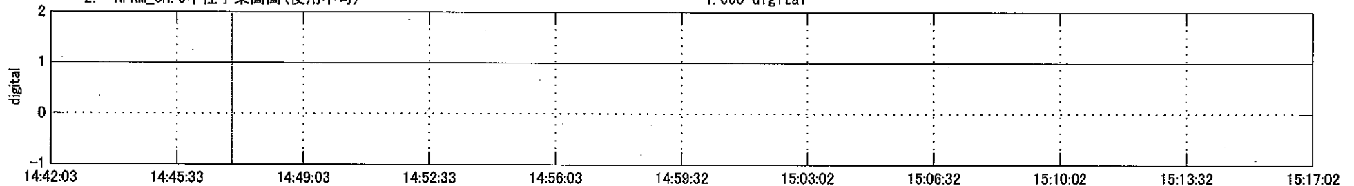
3. APRM_CH. 6中性子束高高(使用不可)
