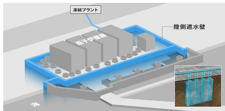
凍土方式の遮水壁施工概要
