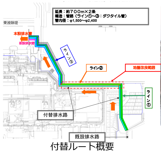
B・C排水路付替工事
