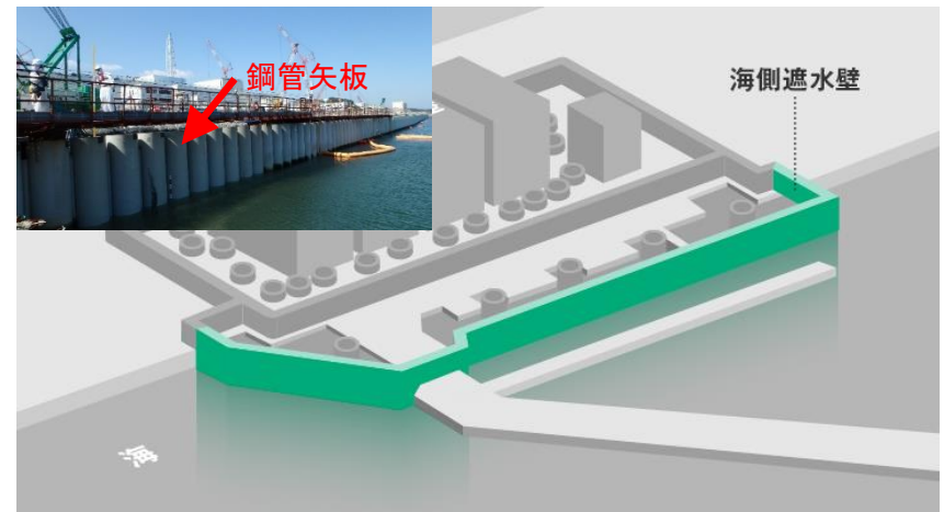
海側遮水壁施工概要
