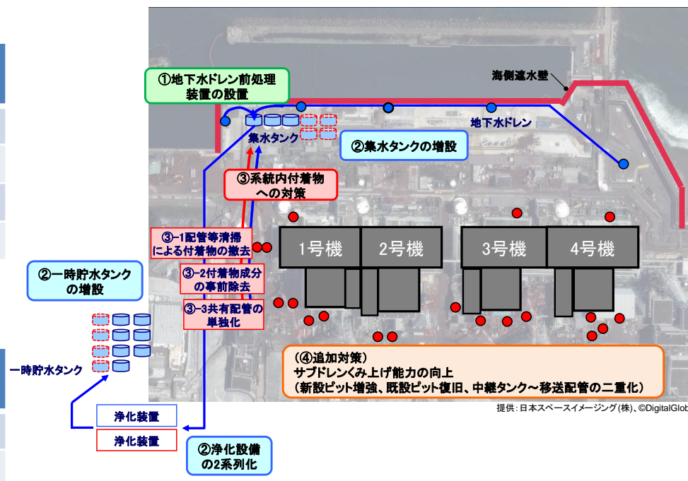
サブドレン他強化対策の概要
