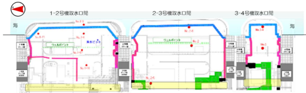
水ガラスによる地盤改良施工箇所
