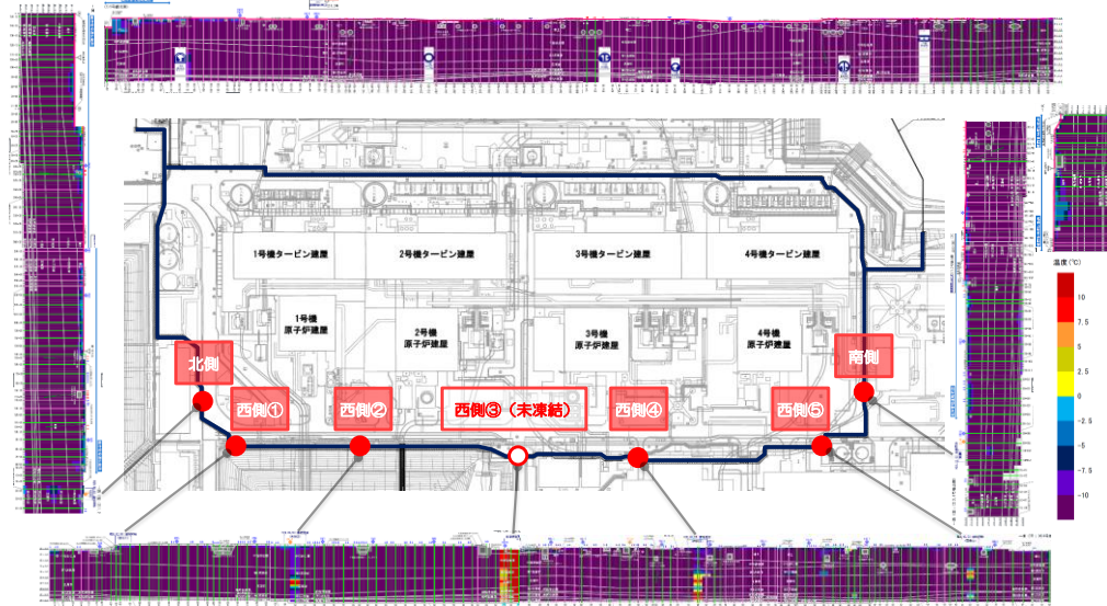
陸側遮水壁凍結状況
