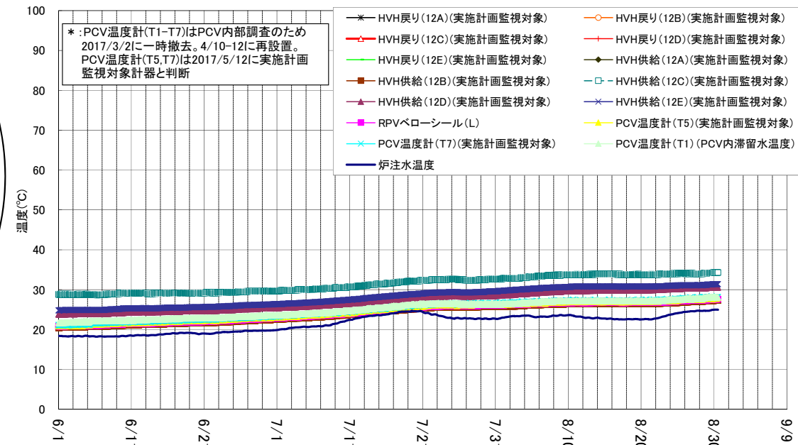
1号機 D/W雰囲気気温度 (6/1~8/30)
