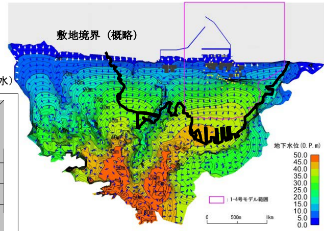
地下水コンター、流向図の解析結果 既存解析モデルの対象範囲
