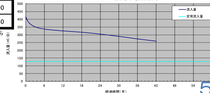
フェーシングの非定常解析結果
