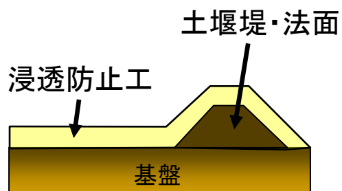
土堰堤・法面方式
