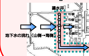
地下水バイパスにより、建屋付近の地下水位を低下させ、建屋への地下水流入を抑制
