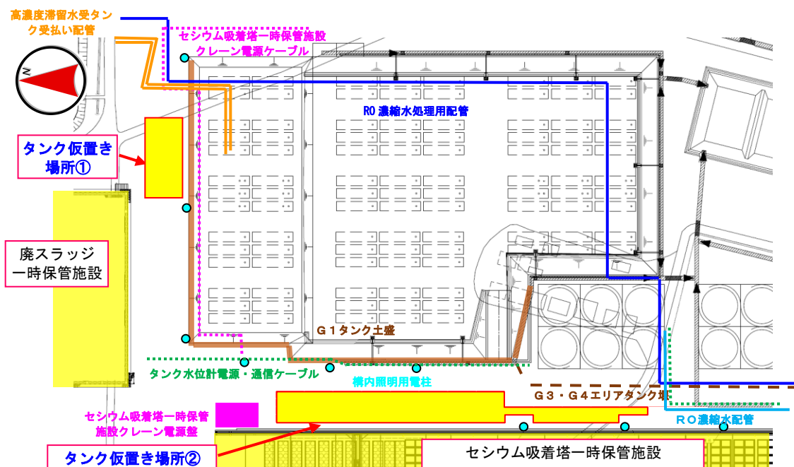
図-4 タンク仮置き場所周辺図
