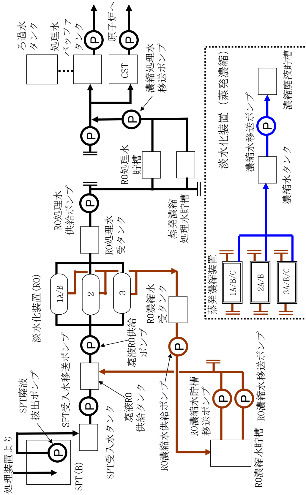
図一七 淡水化装置（逆浸透膜装置，蒸発濃縮装置）の系統構成図
